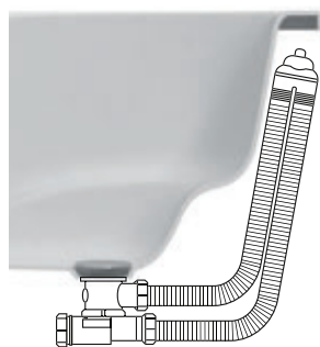
Verdeckte Badewannenablaufgarnitur ohne Überlauf
