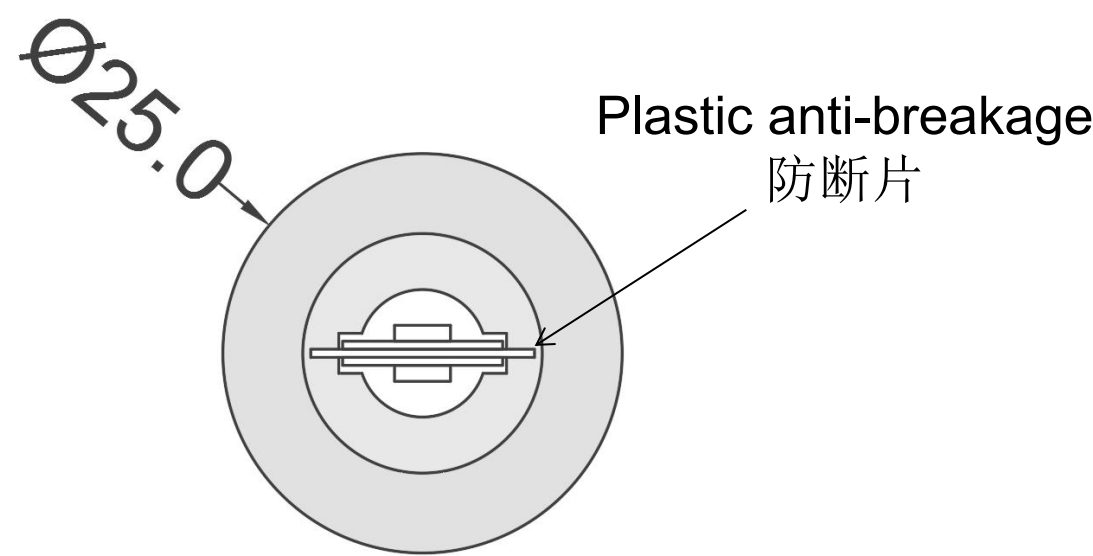
General style 普通款
