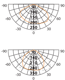
LIGHT INTENSITY CURVES KRZYWE NATEŻENIA ŚWIATŁA LICHTSTÄRKEKURVEN
