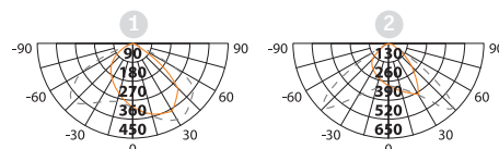
LIGHT INTENSITY CURVES | KRZYWE NATĘŻENIA ŚWIATEŁA | LICHTSTÄRKEKURVEN
