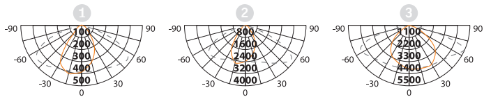
LIGHT INTENSITY CURVES | KRZYWE NATĘŻENIA ŚWIATŁA | LICHTSTÄRKEKURVEN
