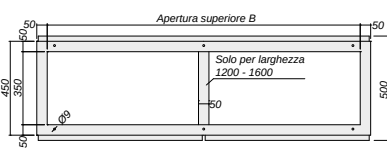
Apertura superiore cassa 1000 - 1200 - 1600
