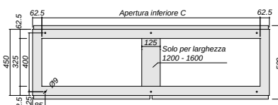
Apertura inferiore cassa 1000 - 1200 - 1600
