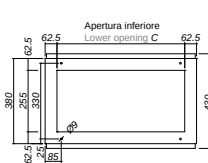
Apertura inferiore cassa Lower opening box 600 - 800
