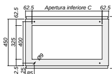
Apertura inferiore cassa 600 - 800
