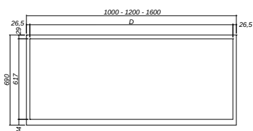
Apertura frontale e posteriore cassa Front and back open box 1000 - 1200 - 1600
