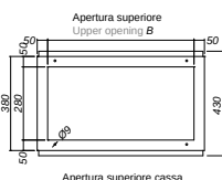
Apertura superiore cassa Upper opening box 600-800
