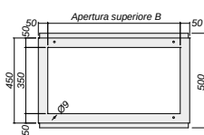
Apertura superiore cassa 600 - 800
