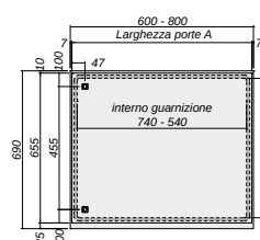
Vista frontale cassa 600 - 800
