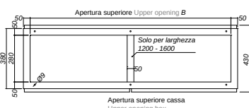
Apertura superiore cassa Upper opening box 1000 - 1200 - 1600
