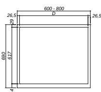
Apertura frontale e posteriore cassa Front and back open box 600 - 800
