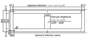
Apertura inferiore cassa Lower opening box 1000 - 1200 - 1600
