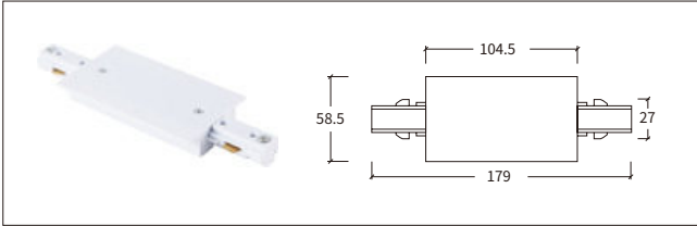
3线A嵌入式 直线连接器 Straight Connector
