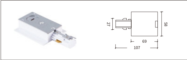
3线A嵌入式 电源连接器-左 Feeder-L
