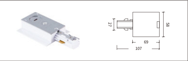
3线A嵌入式 电源连接器-右 Feeder-R
