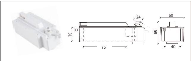
NO: YND-219 2 线短电器箱
