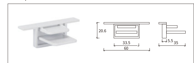
2线嵌入式尾盖 End Cap
