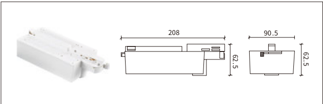
NO: YND-207 2 线大电器箱
