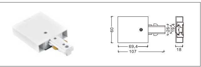
NO: YND-3-H-F 3 线外挂电源头
