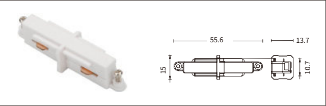
2 线迷你低压导轨条 - 迷你直接驳器
