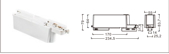
NO: YND-366 配 YND-310 导轨条
