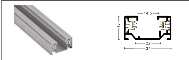
NO: YND B-02 假 3 线导轨条
