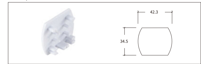
H-01 尾盖 End Cap
