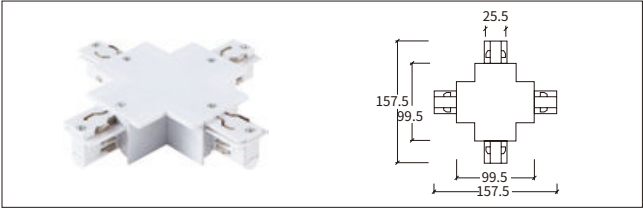
H-03 四线连接器 X-Connector
