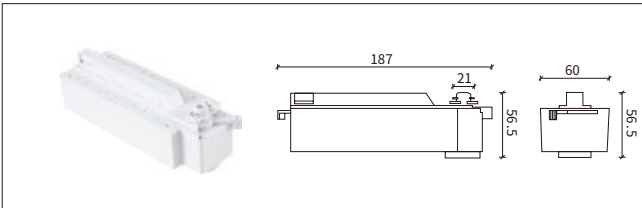
NO: YND-208 2 线小电器箱
