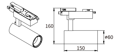
YND-GDT007-60 配电箱 Φ60 Driver Box Φ60
