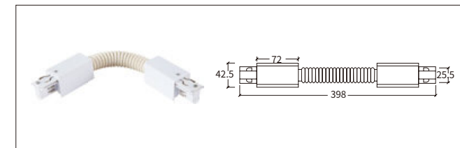
H-02 多角度连接器 (软接) Flexible Connector
