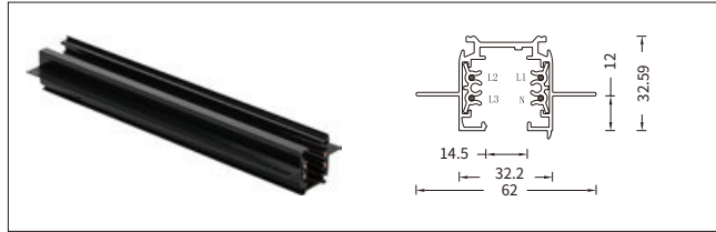
NO: YND-H-041 4线嵌入式导轨
