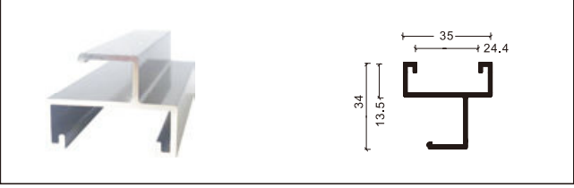
二线、三线外挂导轨挂件
