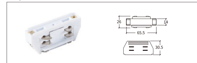
H-01 mini型直线连接器 Straight Connector MINI
