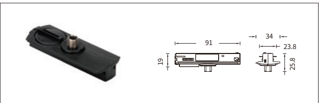
NO: YND-217S 2 线带地线导轨头
