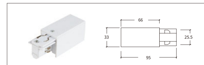
H-02 电源连接器-左 Feeder-L
