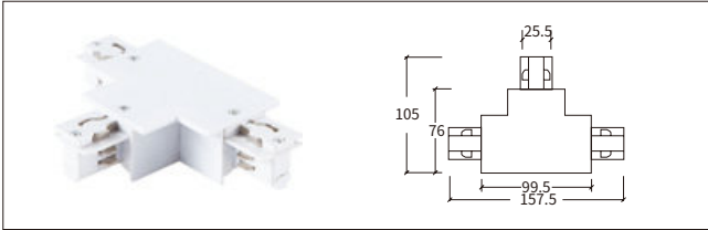
H-03 三向连接器-左 T-Connector-L
