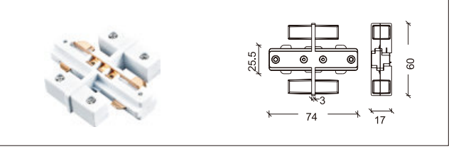
NO: YND-3-H-MINI 3 线挂内接
