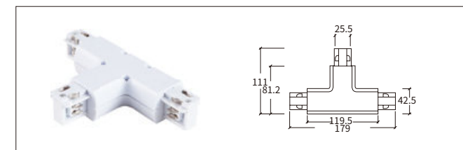
H-01 三向连接器-左 T-Connector-L
