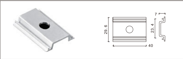
3 线桥架挂件
