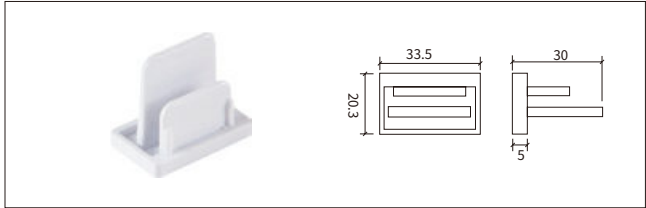
2线 尾盖 End Cap
