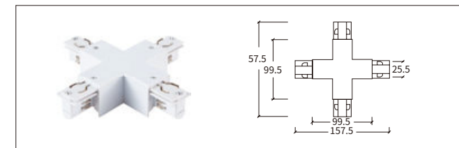
H-02 四向连接器 X-Connector
