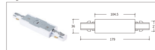
3线A 直线连接器 Straight Connector
