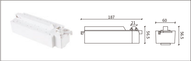
NO: YND-307 3 线小电器箱
