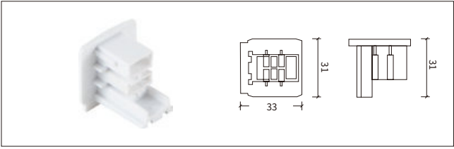
H-05 尾盖 End Cap
