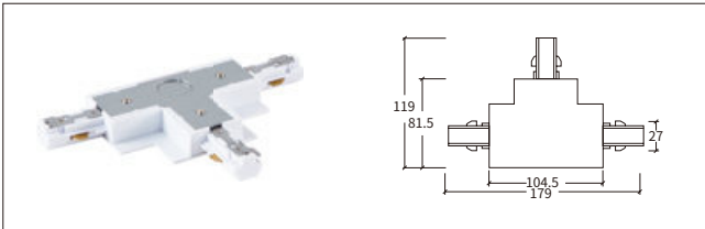
3线A嵌入式 三向连接器-左 T-Connector-L
