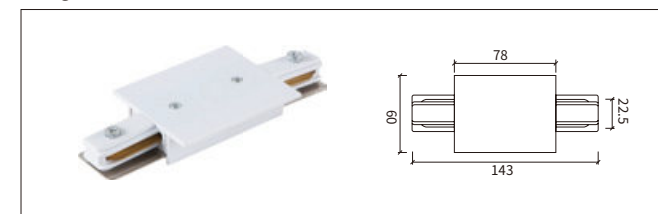
2线嵌入式直线连接器 Straight Connector
