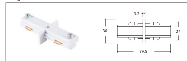
3线A 迷你型直线连接器 Straight Connector MINI
