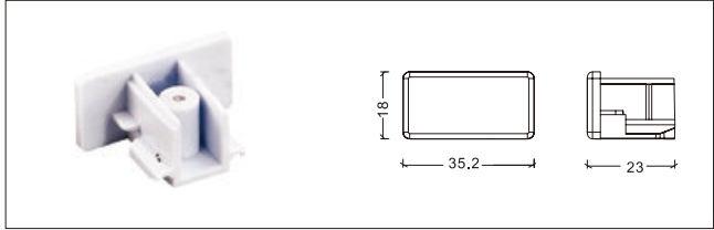
NO: YND B-02-End Cap 假 3 线尾塞
