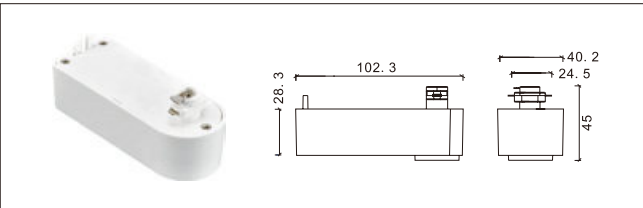
NO: YND-3003 线迷你电器盒
