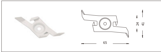
H04 新方型导轨旋转吊挂件
