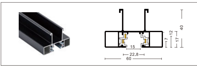
NO: YND-3-H 3 线外挂导轨条
