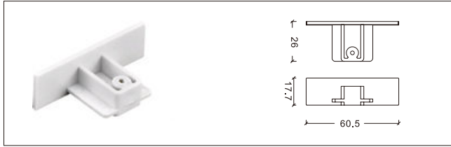
NO: YND-YND-2-H-E 2 线外挂尾塞
