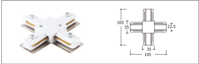
2线 四向连接器 X-Connector
