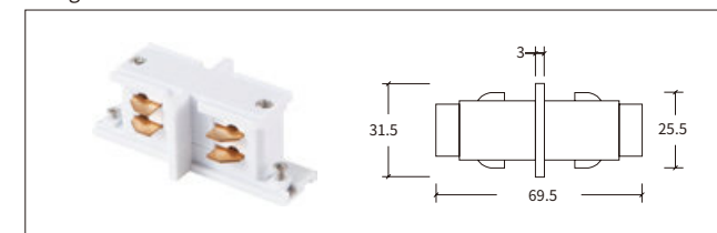
H-04 迷你型直线连接器 Straight Connector MINI
