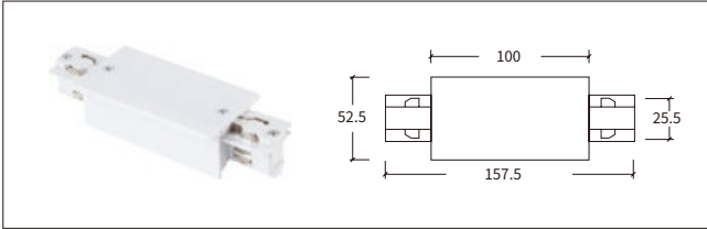
H-03 直线连接器 Straight Connector
