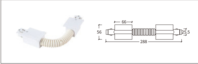
H-03 多角度连接器 (软接) Flexible Connector
