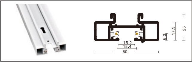
NO: YND-2-H 2 线外挂导轨条
