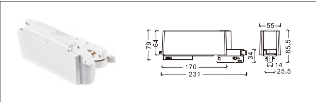
NO: YND-366 配 YND-303 导轨条
