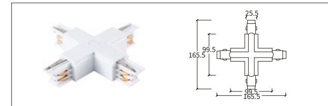
H-04 四向连接器 X-Connector
