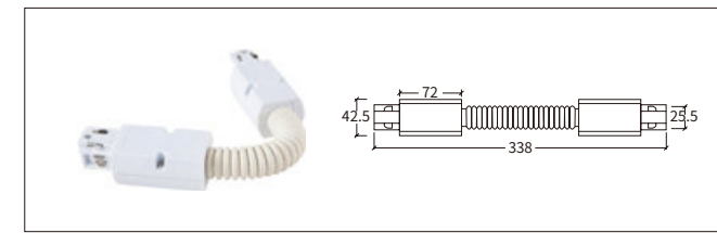
H-01 多角度连接器 (软接) Flexible Connector
