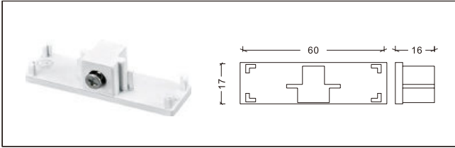
NO: YND-3-H-E 3 线外挂尾塞
