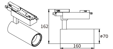
YND-GDT007-70 配电箱 Φ70 Driver Box Φ70
