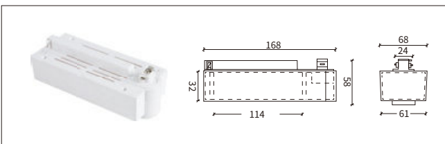
NO: YND-314 3 线简易电器箱
