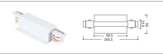
H-05 直线连接器 Straight Connector
