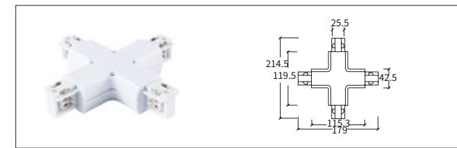
H-01 四向连接器 X-Connector
