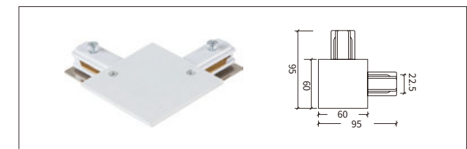
2线嵌入式L型连接器 L-Connector
