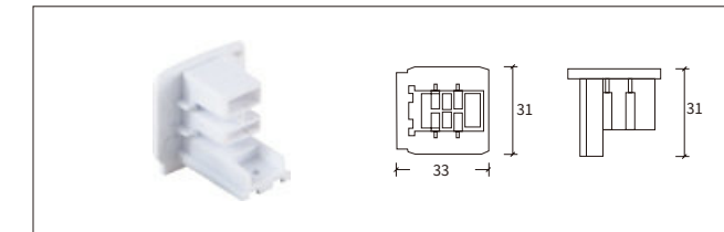
H-04 尾盖 End Cap
