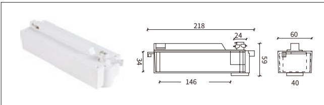
NO: YND-311 3 线长电器箱
