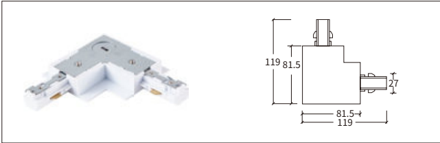
3线A嵌入式 L型连接器-左 L-Connector-L
