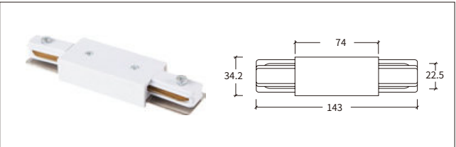
2线 直线连接器 Straight Connector
