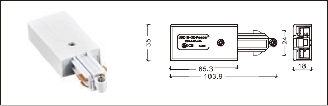
NO: YND B-02-Feeder 假 3 线电源头
