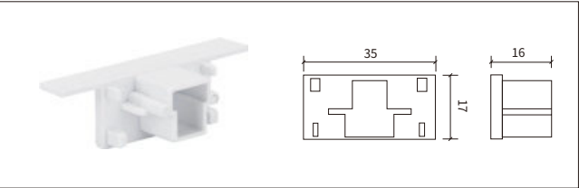
3线A 尾盖 End Cap
