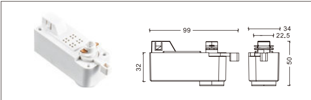
NO: YND-2112 线小电源盒
