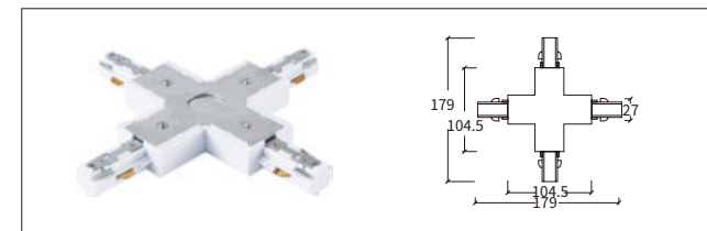
3线A 四向连接器 X-Connector
