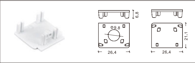
NO: 2 线迷你导轨条尾盖
