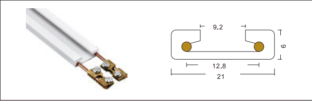
NO: YND-2R-2RO 2 线软导轨
