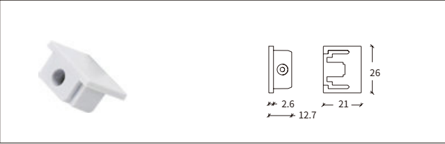
2 线低压导轨尾塞
