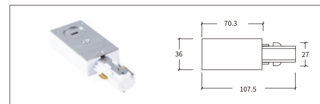
3线A 电源连接器-左 Feeder-L
