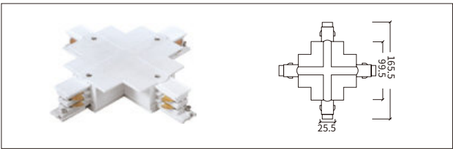
H-05 四向连接器 X-Connector
