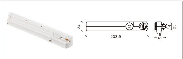
NO: YND-333 3 线长款电源盒
