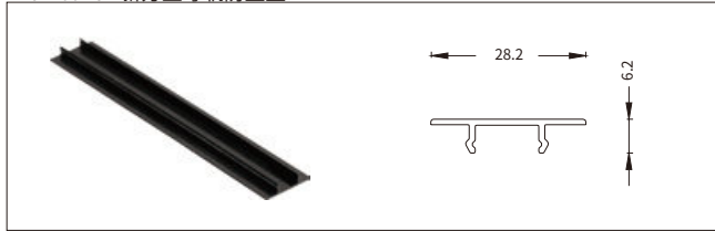
H-04-cover 新方型导轨防尘盖
