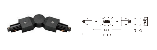
NO: YND B-02-K 假三线任意角度接驳 (硬接)
