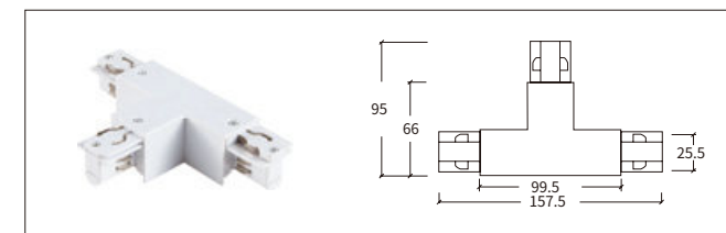
H-02 三向连接器-左 T-Connector-L
