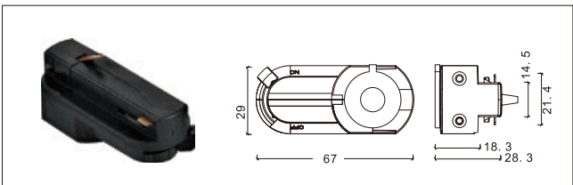
NO: YND-271小二线
