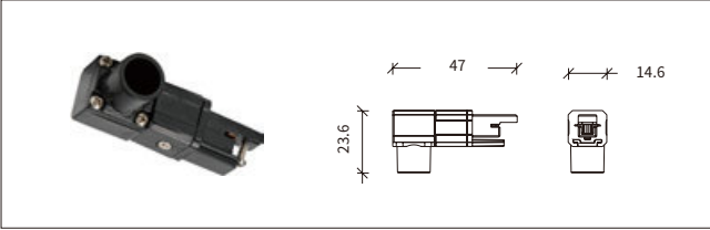
可旋转电源头
