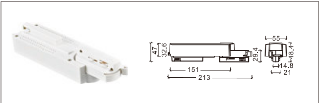
NO: YND-269 配 YND-209 导轨条
