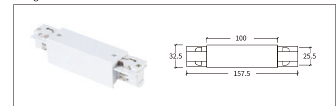
H-02 直线连接器 Straight Connector
