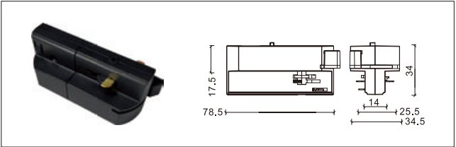
NO: YND-303-S 三线简易型
