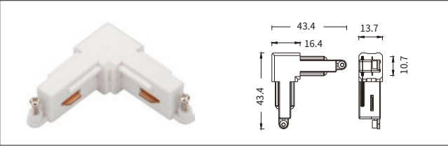
2 线迷你低压导轨条 -L 型接驳器
