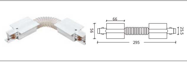
H-05 多角度连接器 (软接) Flexible Connector
