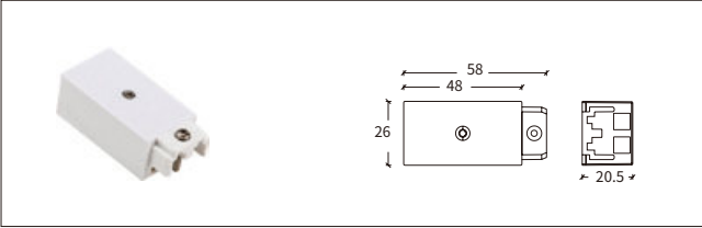
2 线低压导轨电源头
