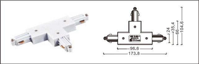
NO: YND B-02-T 假3线T接
