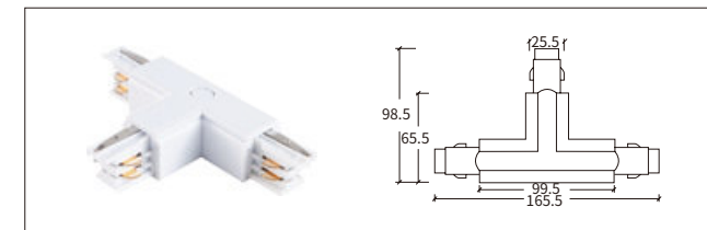
H-04 三向连接器-左 T-Connector-L
