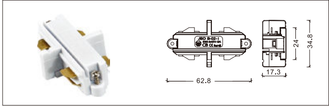
NO: YND B-02-I-NIMI 假 3 线内接
