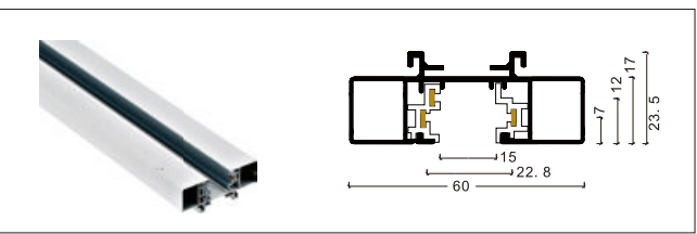
3 线外挂导轨条 (短款)
