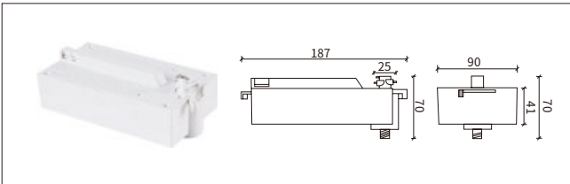
NO: YND-305 3 线一体电器箱
