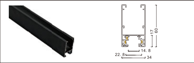
3 线桥架导轨条
