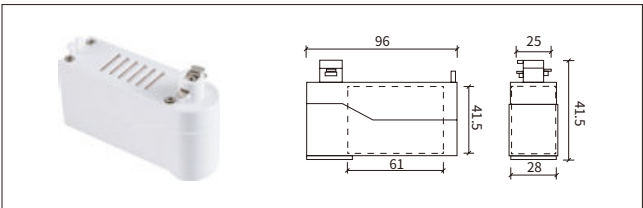
NO: YND-313 3 线筒体电器箱
