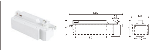
NO: YND-306 3 线短电器箱
