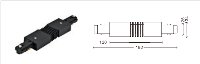
3线 短软连接器 Connector
