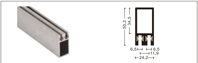
NO: P-03-R 展柜式导轨条
