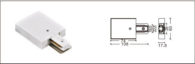
NO: YND-2-H-F 2 线外挂电源头
