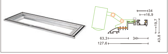
NO: 隐藏式射灯支架
