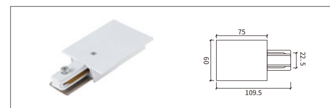
2线嵌入式 电源接头 Feeder
