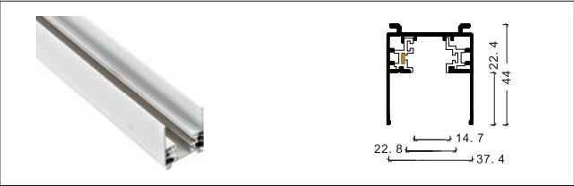
3 线高边导轨条
