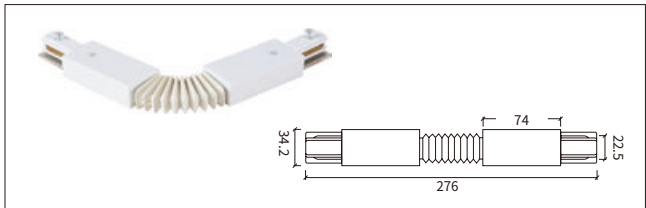
2线 多角度连接器(软接) Flexible Connector
