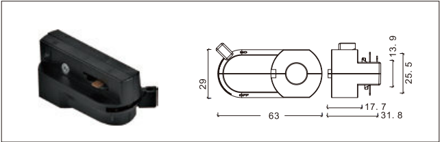
NO: YND-371 小三线
