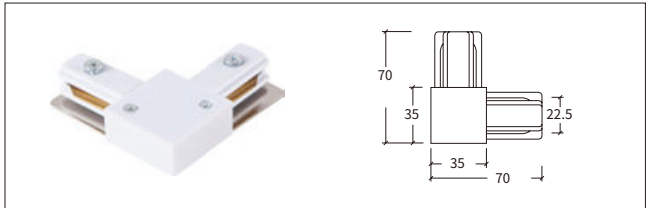
2线L型连接器 L-Connector
