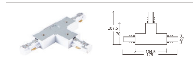
3线A 三向连接器-左 T-Connector-L
