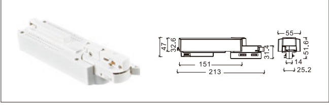
NO: YND-369 配 YND-303 导轨条
