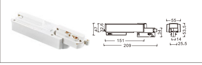
NO: YND-369 配 YND-310 导轨条
