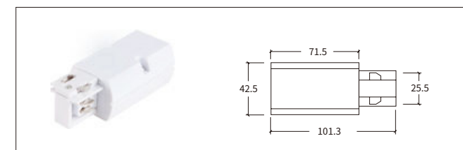
H-01 电源连接器-左 Feeder-L
