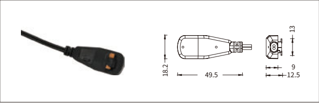
一体取电头 (软导轨)
