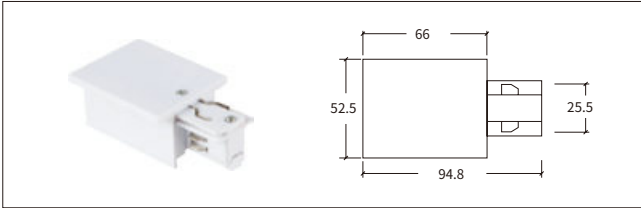
H-03 电源连接器-左 Feeder-L
