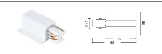
H-05 电源连接器-左 Feeder-L
