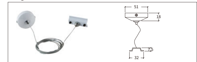
H-02 四线吊绳挂件 Fitting
