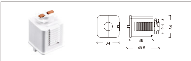
NO: J210 日本 2 线导轨头
