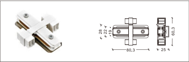
NO: YND-2-H-I 2 线外挂内接
