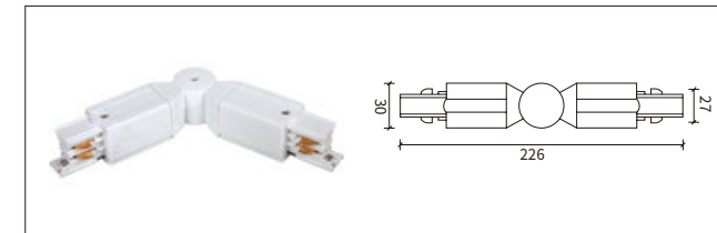
H-04 任意角度连接器 Flexible Connector
