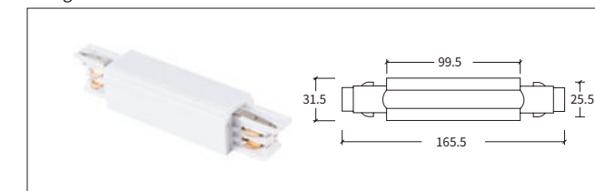
H-04 直线连接器 Straight Connector
