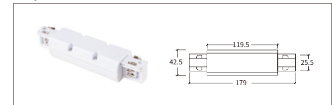
H-01 直线连接器 Straight Connector
