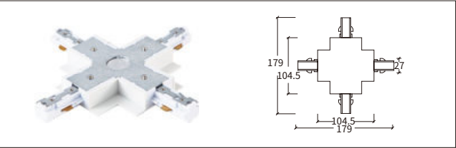
3线A嵌入式 四向连接器 X-Connector
