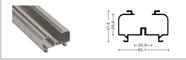
NO: 导轨条铝支架
