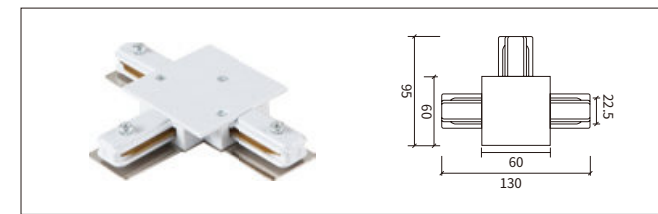
2线嵌入式三向连接器 T-Connector
