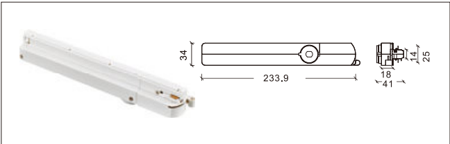
NO: YND-324 3 线长款电源盒 (手柄)
