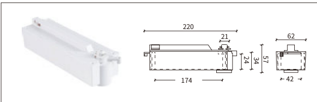
NO: YND-215 2 线长电器箱
