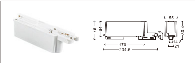
NO: YND-266 配 YND-209 导轨条
