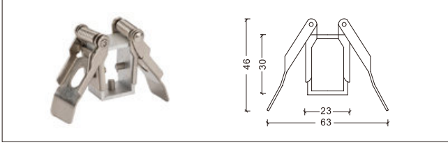
NO: 导轨夹
