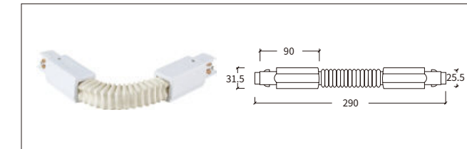
H-04 多角度连接器 (软接) Flexible Connector
