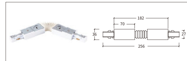
3线A 多角度连接器(软接) Flexible Connector
