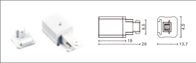
NO: 2 线迷你导轨电源头
