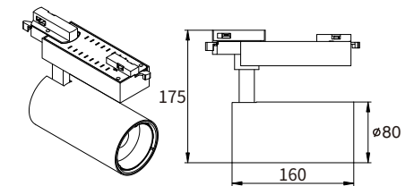
YND-GDT007-80 配电箱 Φ80 Driver Box Φ80
