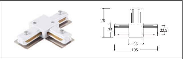
2线 三向连接器 T-Connector
