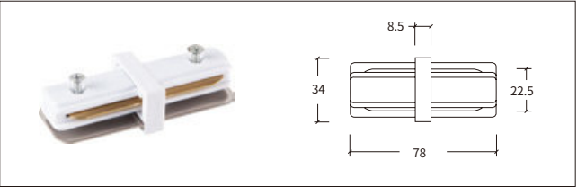
2线 内接 Straight Connector MINI
