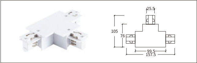
H-03 三向连接器-右 T-Connector-R
