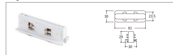
H-02 mini型直线连接器 Straight Connector MINI
