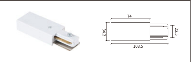
2线A 电源接头 Feeder
