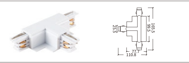
H-05 三向连接器-左 T-Connector-L
