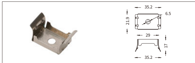
H-04-fitting 新方型导轨弹性吊挂件
