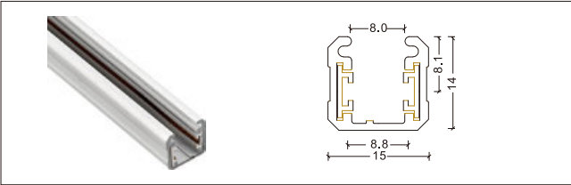
NO: 2 线迷你导轨条
