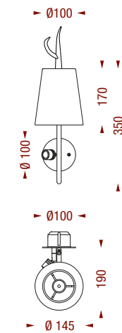
Z99-DEE-W1-L (Leseleuchte links)
