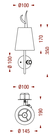
Z99-DEE-W1-R (Leseleuchte rechts)
