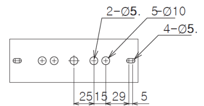
(Bracket)
