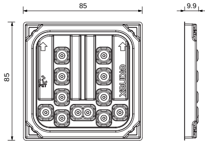
Dimensions [mm] - serie 20venti Deep
