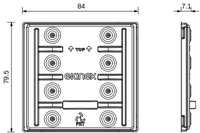
Dimensions [mm] - serie 20venti Deep
