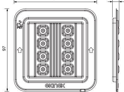
Dimensions [mm] - serie 71 Deep
