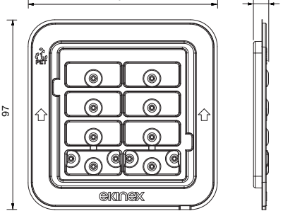
Dimensions [mm] - serie 20venti Surface
