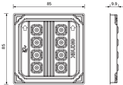
Dimensions [mm] - serie 71 Deep
