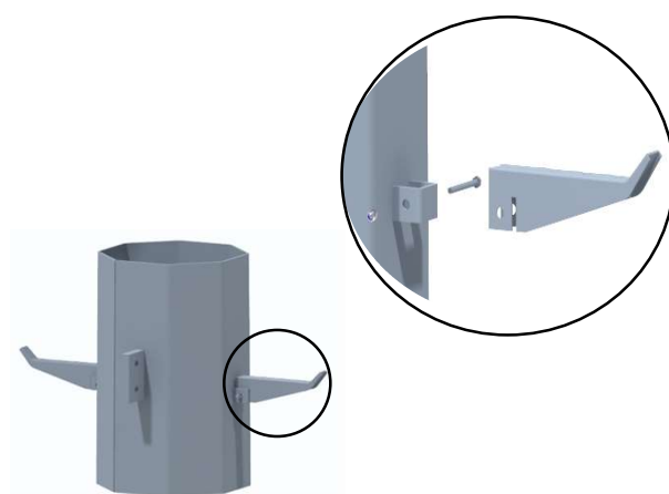
Abnehmbare Steigsprosse
