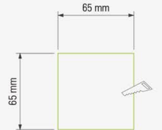
TAVAN KESİM ÖLÇÜSÜ CEILING CUT-OUT SIZE
