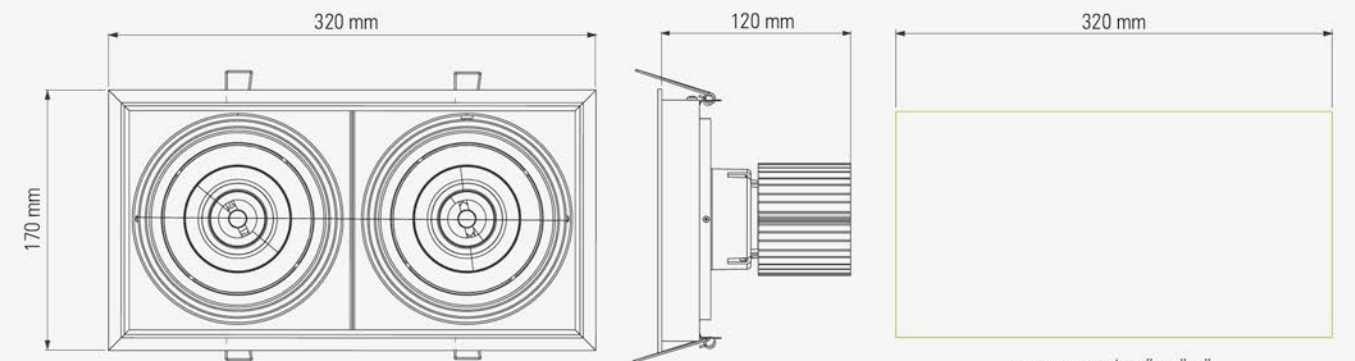
TAVAN KESİM ÖLÇÜSÜ CEILING CUT-OUT SIZE
