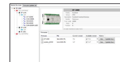
Firmware Updater
