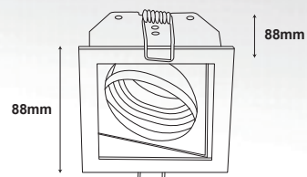
FDAD-S2
