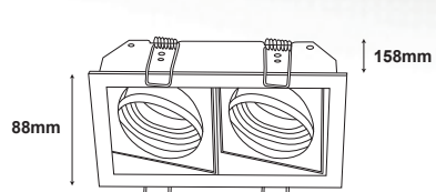
FDAD-S1
