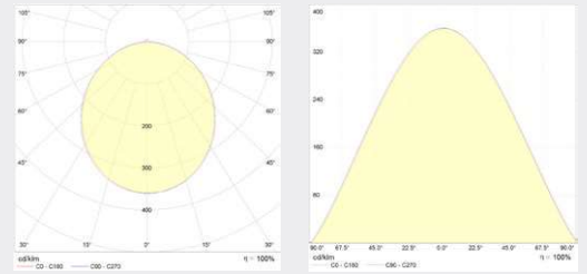
Kutup Eğrisi Polar Curve
