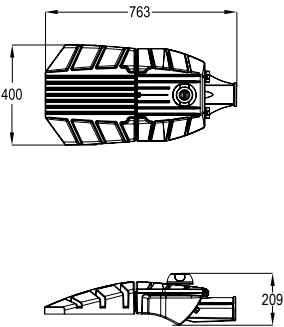
TRIMAX R1 - Post Top
