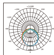
VLOE-215T Photometric
