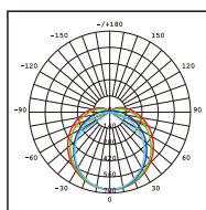
VLOE-115T Photometric
