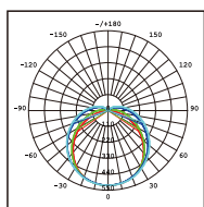
VLOE-112T Photometric
