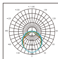
VLOE-212T Photometric
