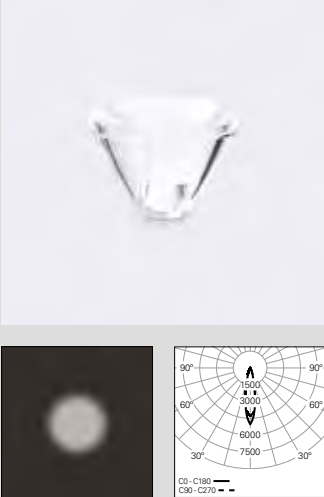
4.1. 14° lens
