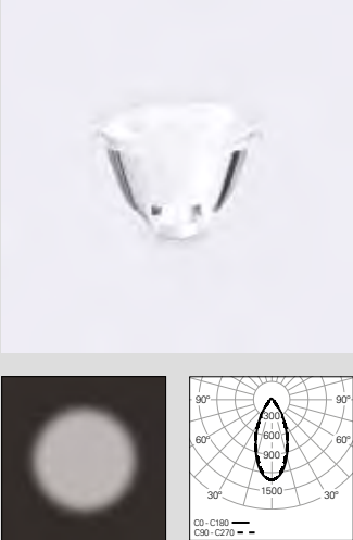
4.2. 47° lens
