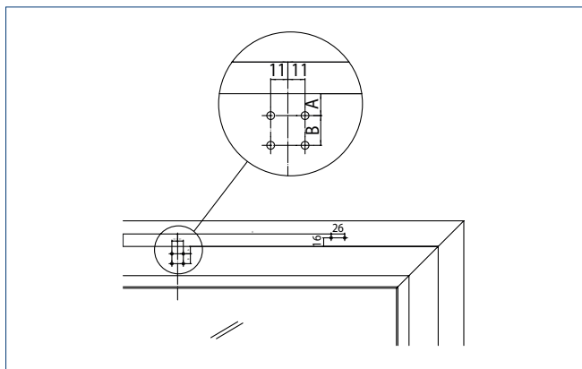
Rahmenmontage EINWÄRTS
