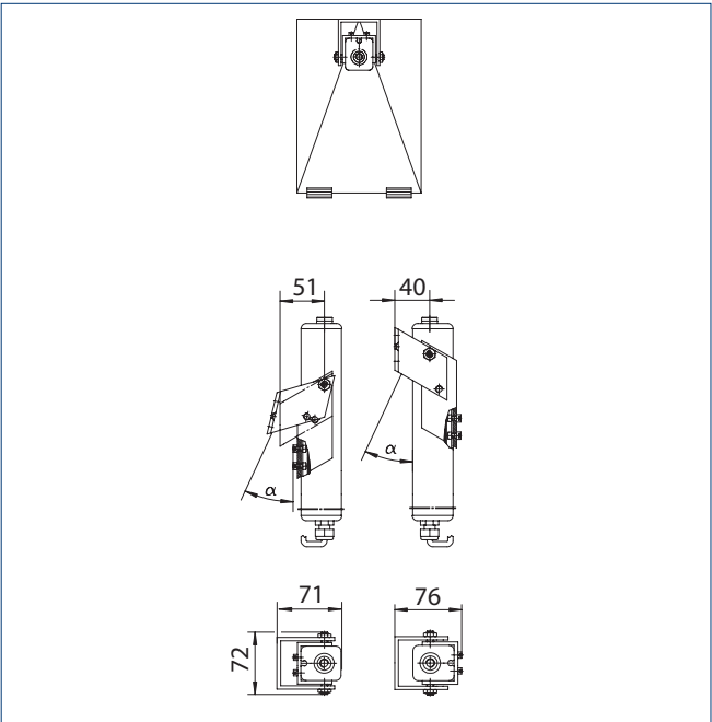
Standardkonsole
