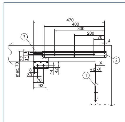
Montage Konsolen
