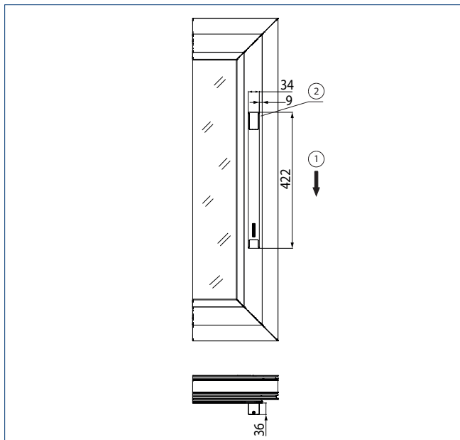
Platzbedarf Flügelmontage
