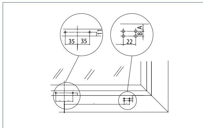
Flügelmontage EINWÄRTS
