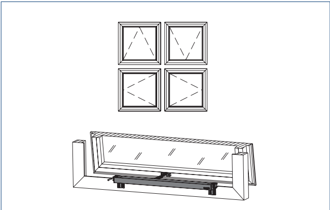
Konsolensatz B
