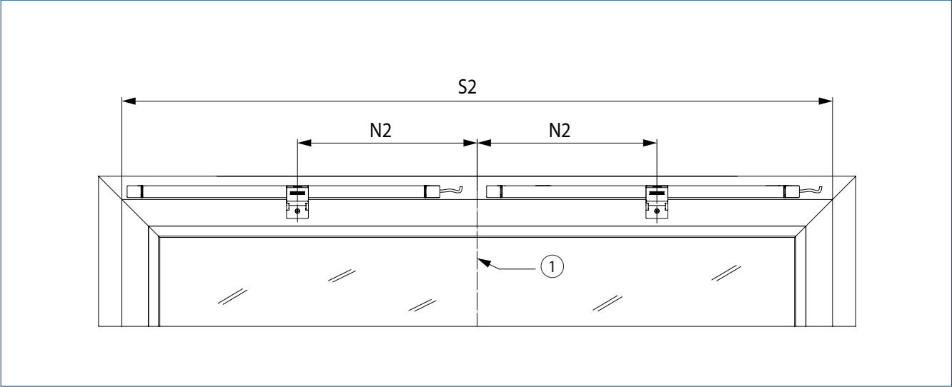
Maße für S2 und N2 siehe Tabelle 1 = Mitte Fenster
