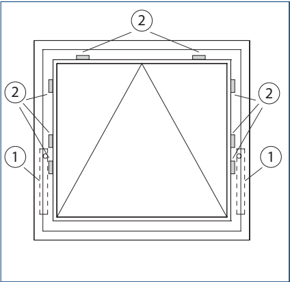
1 = Mögliche Montagevarianten E 905 / E 906 I 2 = Mögliche Verriegelungspunkte über Zentralverschluss
