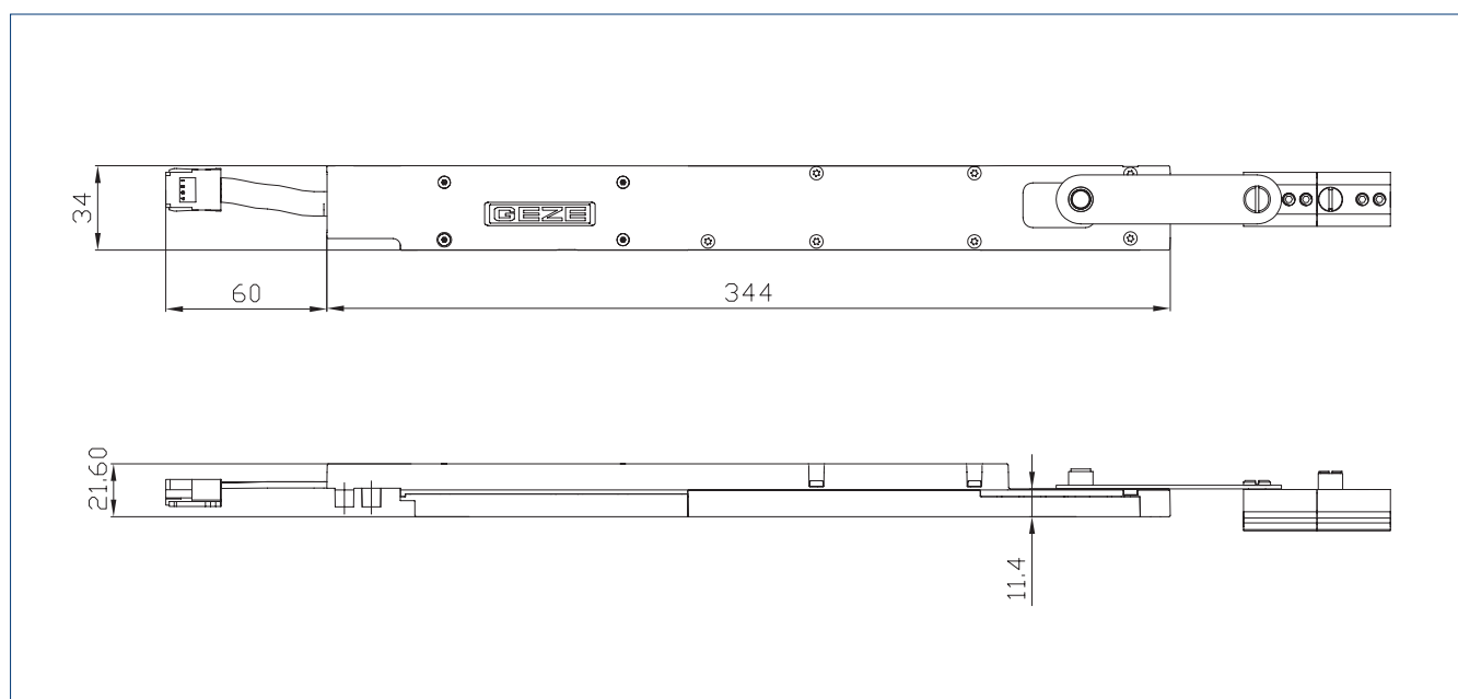
Abbildung spiegelsymmetrisch für GEZE E 906
