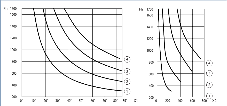
X1 = Öffnungswinkel | X2 = Platzbedarf für Schwenkung (mm) | Fh = Flügelhöhe (mm) | 1 = Hub 300 | 2 = Hub 500 | 3 = Hub 750 | 4 = Hub 1000
