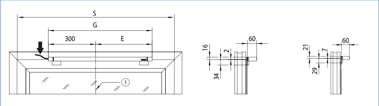
Maße für E, G und S siehe Tabelle | 1 = Mitte Fenster
