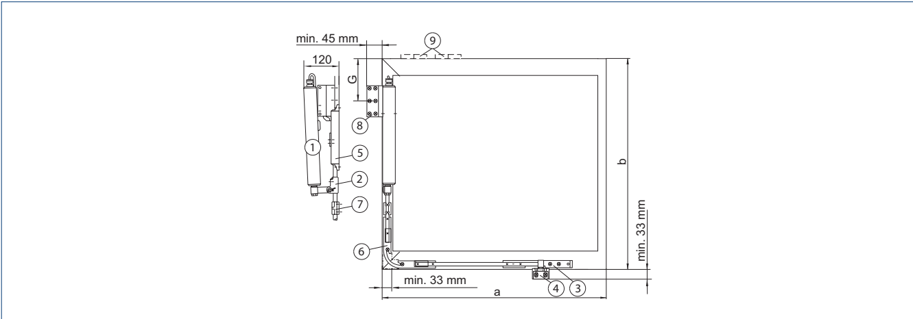
Anschlagmaße G und E siehe Tabelle a = Flügelbreite | b = Flügelhöhe | 1 = Elektrospindelantrieb E 350 | 2 = Stangenübertragung | 3 = Zusatzverriegelung OL 320 | 4 = Zusatzwinkel vollständig | 5 = Entriegelungsfeder | 6 = Eckumlenkung OL 320 | 7 = Stangenführung OL 320 | 8 = Rahmenwinkel | 9 = 2 Bänder auf der Antriebsseite (bauseits vorzusehen)
