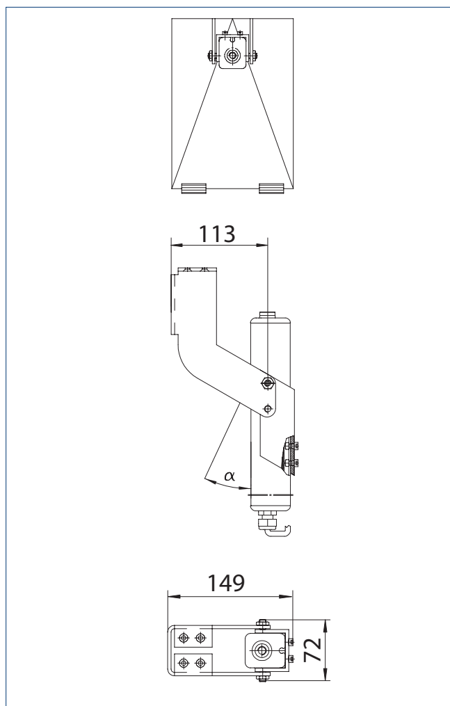
Konsole EINWÄRTS
