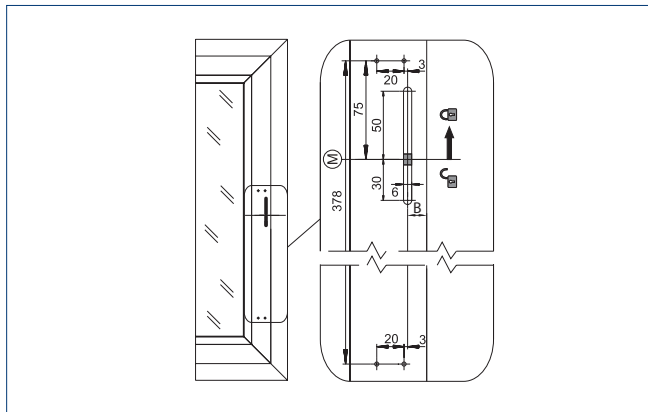
Montagemasse Flügelmontage
