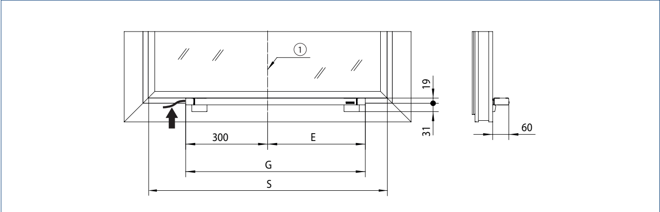
Maße für E, G und S siehe Tabelle | 1 = Mitte Fenster
