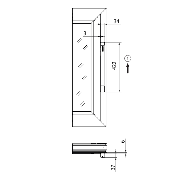
Platzbedarf Rahmenmontage
