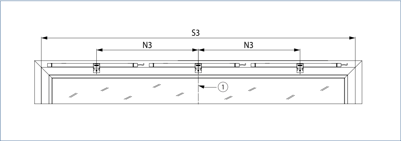
Maße für S3 und N3 siehe Tabelle 1 = Mitte Fenster
