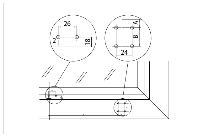
Flügelmontage EINWÄRTS
