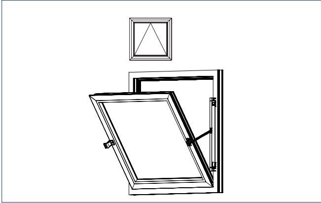
Konsolensatz A
