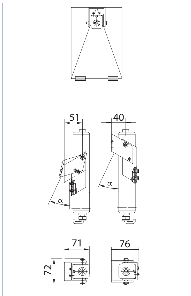
Standardkonsole
