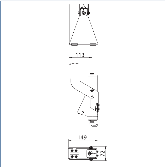
Konsole EINWÄRTS
