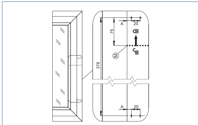
Montagemasse Rahmenmontage
