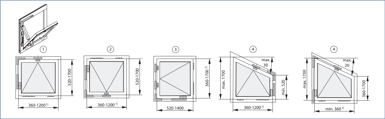
Alle Angaben in mm 1 = Kippfenster | 2 = Klappfenster | 3 = Drehfenster | 4 = Schrägfenster Kipp | 1) Für Kunststofffenster Solo max. 800 mm
