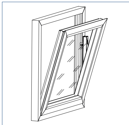
Rahmenmontage
