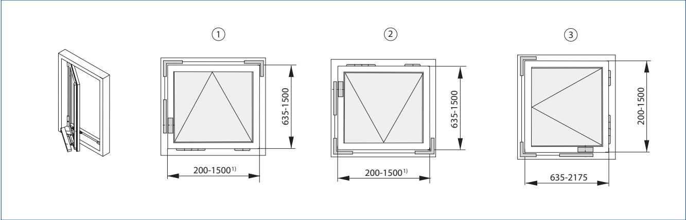
Alle Angaben in mm 1 = Kippfenster | 2 = Klappfenster | 3 = Drehfenster | 1) Für Kunststofffenster Solo max. 800 mm
