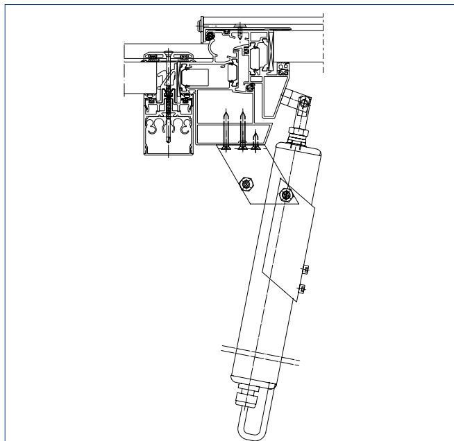
Standardkonsole E 250 NT / E 350 N, inkl. Standard-Flügelbock (Id.Nr. 019032)
