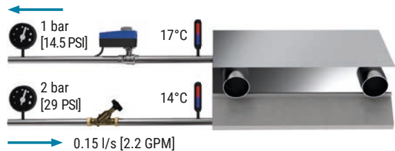
Abb. 89: Kühlbalken mit einem druckabhängigen Ventil.
