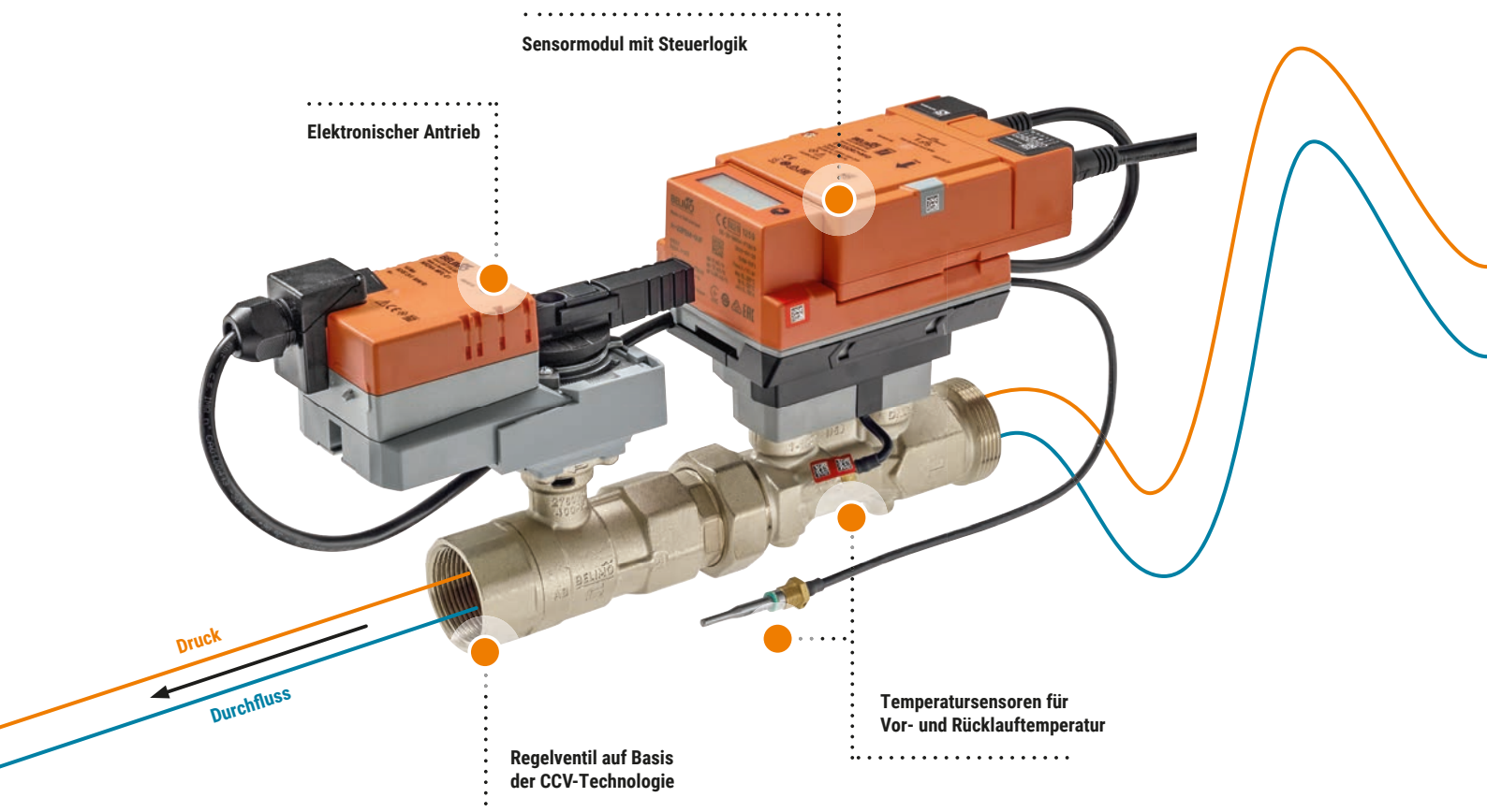
Abb. 12: Elektronisches PI-Ventil von Belimo, z.B. ein EPIV.
