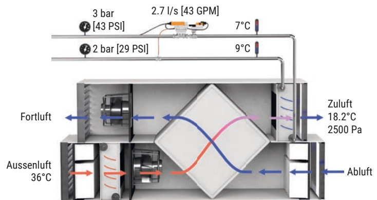
Abb. 56: RLT-Gerät ohne Ventilüberlauf.
