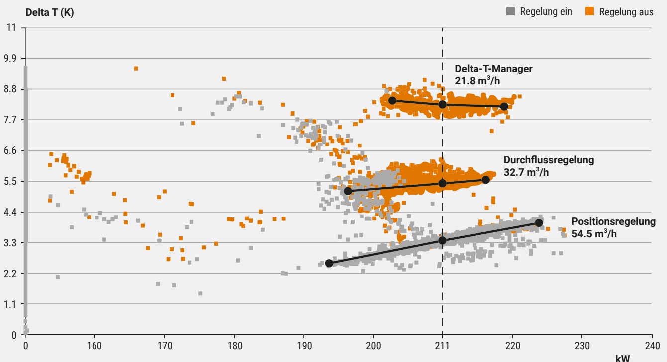
Abb. 31: Betriebsbedingungen (Delta T und Last) des Ventils in verschiedenen Regelmodi.
