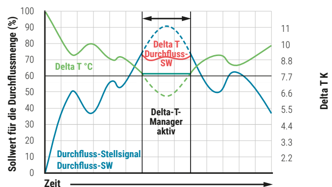
Abb. 30: Der Delta-T-Manager erkennt ein niedriges Delta T, wird aktiv und reduziert den Durchfluss, um das minimale Delta T zu gewährleisten.
