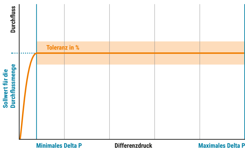
Abb. 75: Dynamischer Abgleich einer FCU.
