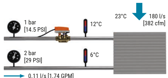
Abb. 78: FCU bei Auslegungsbetrieb.
