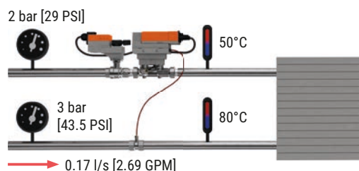
Abb. 100: FCU, mit BMS-korrigiertem Heizsollwert und erforderlichlichem Durchfluss.
