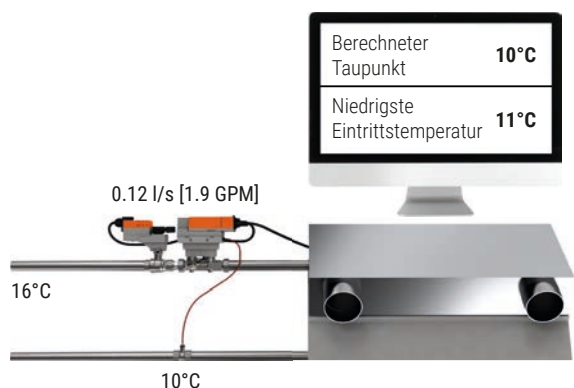
Abb. 92: Kühlbalken mit einem Energieventil, wobei das BMS den Taupunkt anhand der Daten eines Raumsensors berechnet.
