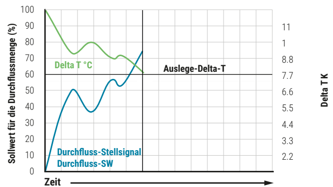
Abb. 28: Wenn der Bedarf steigt und sich der Durchfluss ändert, beginnt das tatsächliche Delta T zu sinken.
