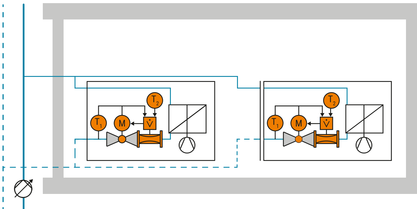
Abb. 74: Typische Gebläsekonvektoranwendung in einem einzigen Raum, mit einem Belimo Energy Valve™ pro Gebläsekonvektor.
