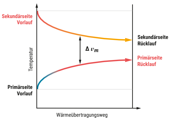
Abb. 63: \Delta \vartheta_m durchschnittliche Differenztemperatur bei Gleichstrom.
