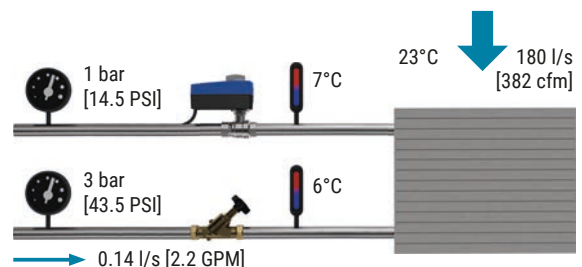
Abb. 77: FCU mit überlaufendem Ventil.
