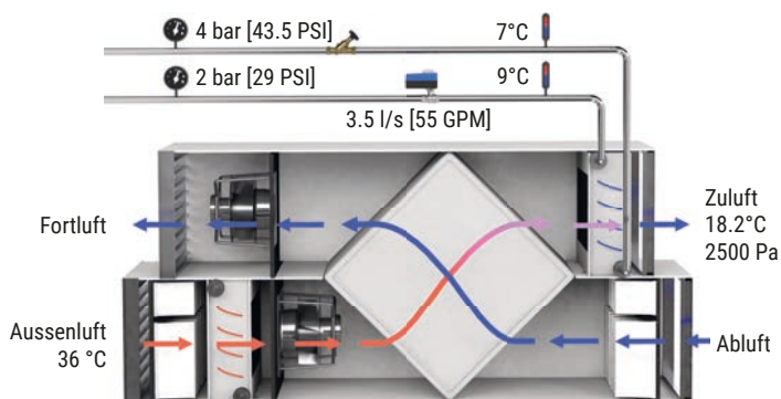
Abb. 54: RLT-Gerät mit überlaufendem Ventil.
