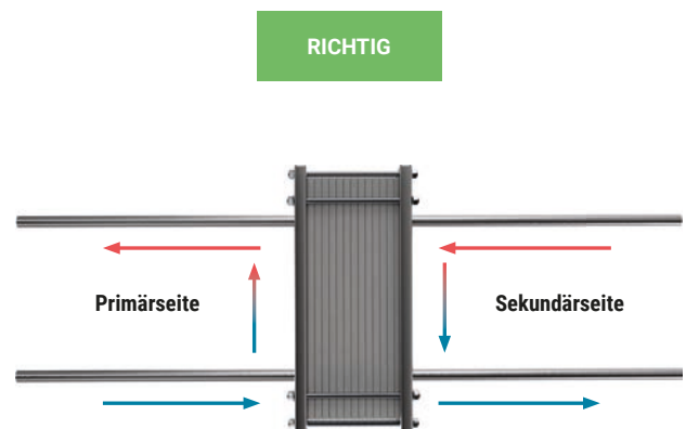
Abb. 64: Kühlungsübergabestation im Gegenstrom angeschlossen.
