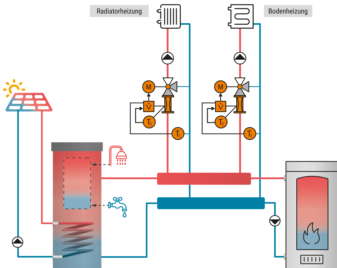
Abb. 115: Typisches Hydraulikschema einer Zentralheizungsanlage, die mehrere alternative und erneuerbare Energiequellen kombiniert.
