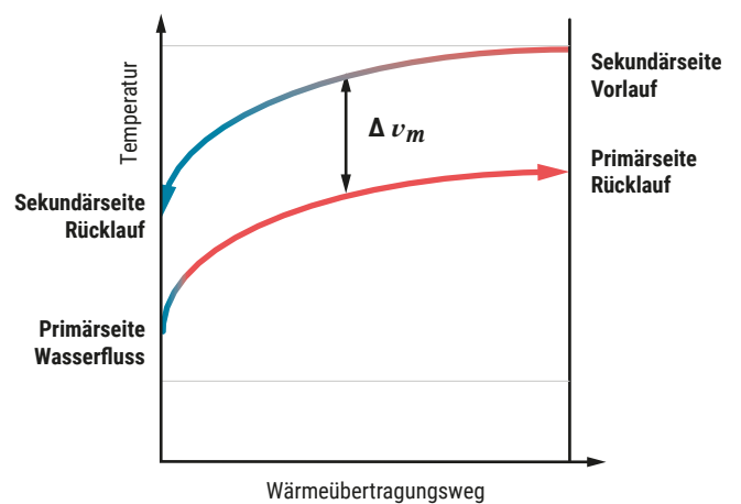
Abb. 65: \Delta \vartheta_m mittlere Differenztemperatur bei Gegenstrom.
