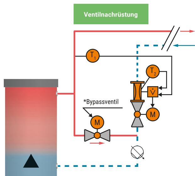
Abb. 117: Ein nicht kondensierender Kessel, der mit einem luftblasendichten Bypassventil und einem Energieventil nachgerüstet wurde.
