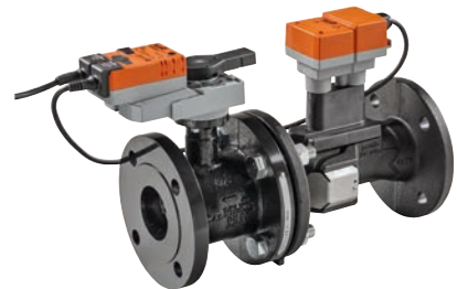
Abb. 3: EPIV
