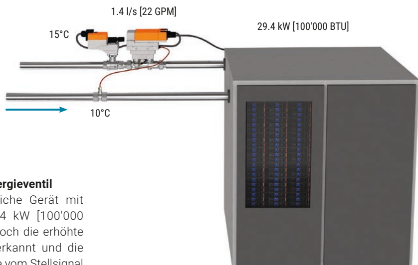
Abb. 112: CRAC-Gerät mit höherer Vorlauftemperatur, um Energie zu sparen.
