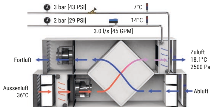
Abb. 53: RLT bei Auslegungsbetrieb.
