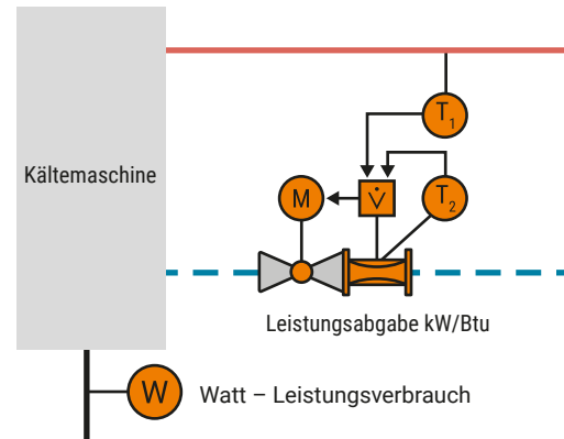
Abb. 120: Kältemaschine mit Kühlkreislauf.
