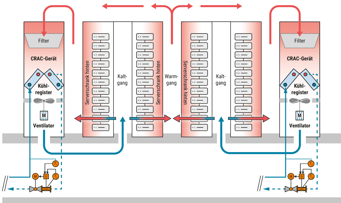
Abb. 110: Schema eines CRAC-Geräts, einschliesslich des Luftstroms zu/von den Racks.
