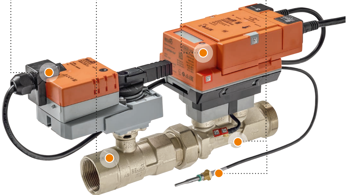
Abb. 21: Die Komponenten des Belimo Energy Valve™.
