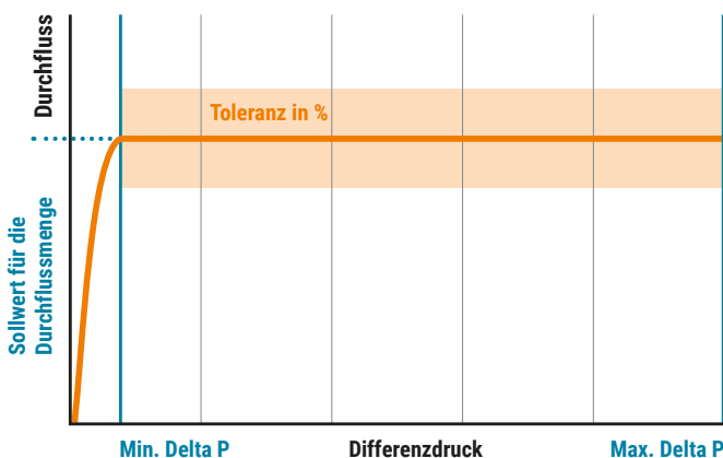
Abb. 85: Dynamischer Abgleich eines Kühlbalkens.
