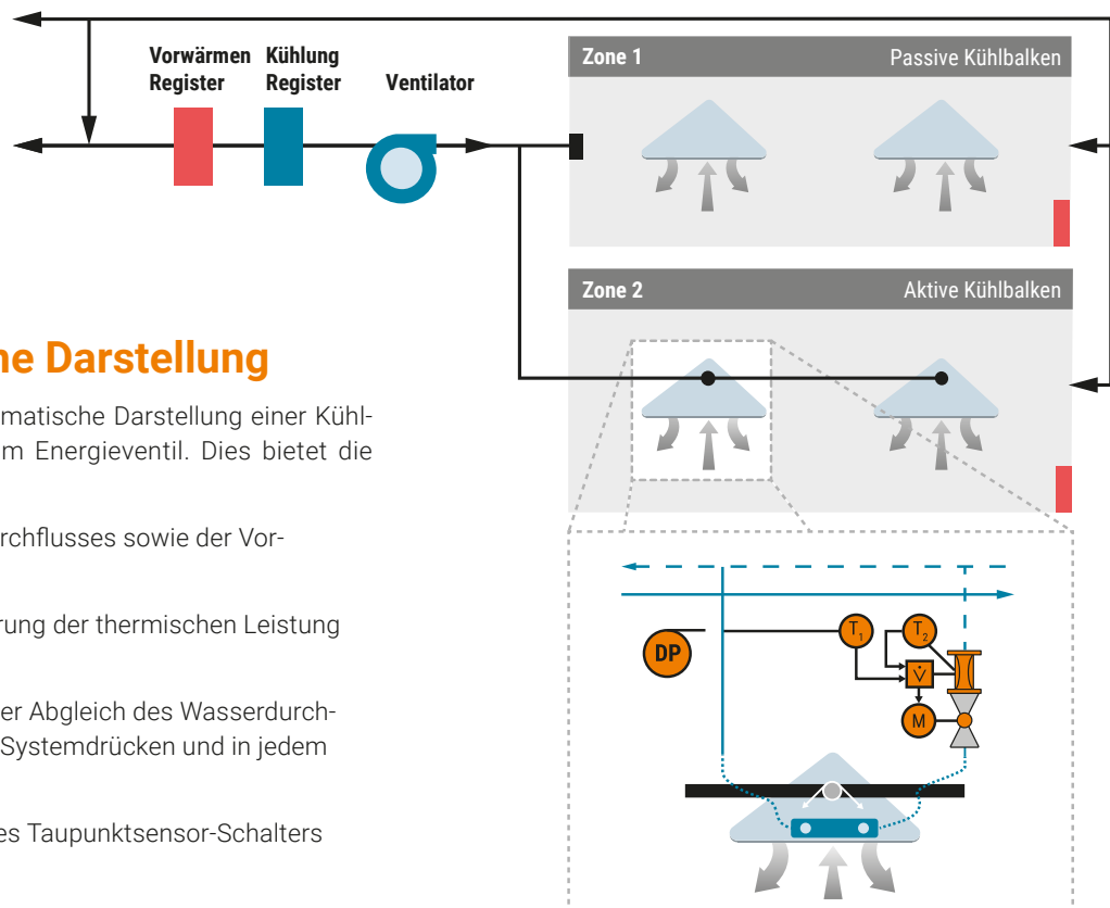
Abb. 84: Kühlbalken in einer Mehrzonenanlage.
