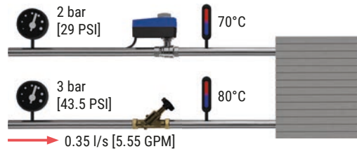
Abb. 97: FCU im Heizbetrieb.
