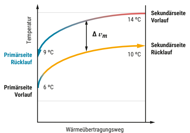
Abb. 69: \Delta v_m mittlere Differenztemperatur bei Sättigung.
