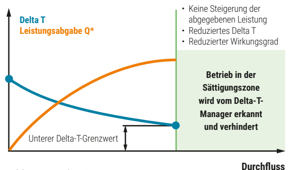
Abb. 107: Delta-T-Manager
