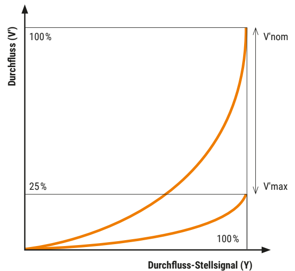
Abb. 23: Durchflusskennlinie in Bezug auf das Durchfluss-Stellsignal.
