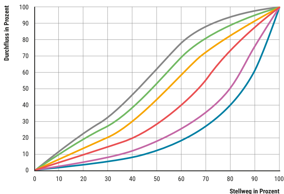
Abb. 22: Die Verzerrung der Kennlinie, die auftreten kann, wenn das Ventil in der Positionsregelung belassen wird.
