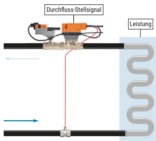
Abb. 25: Leistungsregelung der Energiezufuhr zu einem Verbraucher.
