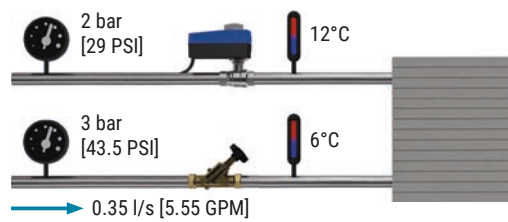
Abb. 96: FCU im Kühlbetrieb.
