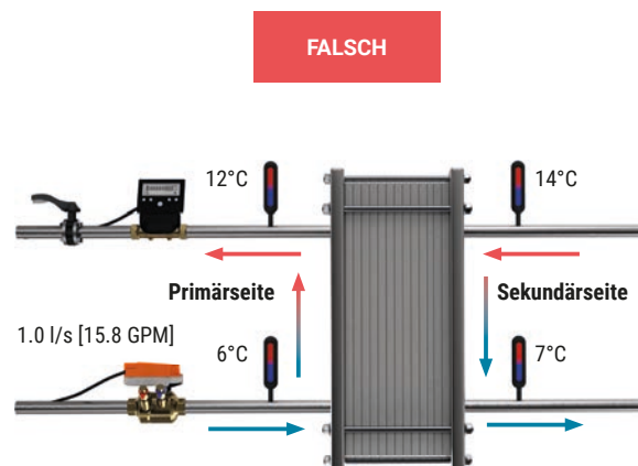
Abb. 70: Dynamischer Abgleich.
