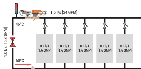
Abb. 105: Mit einem Energy Valve können sowohl undichte Kurzhubventile als auch ein offener Bypass eindeutig identifiziert werden.
