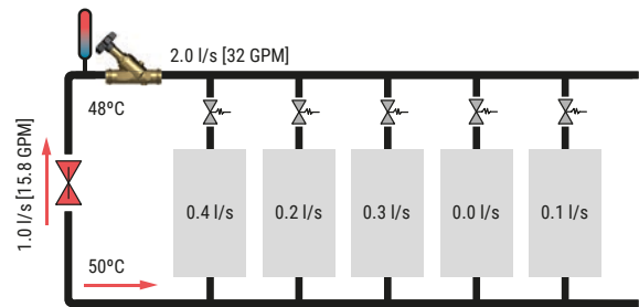
Abb. 104: Ein versehentlich geöffnetes Bypassventil wird möglicherweise erst nach Wochen, Monaten oder sogar Jahren entdeckt.
