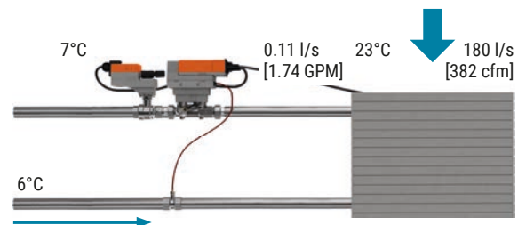
Abb. 79: FCU ohne zu hohe Wassermenge.
