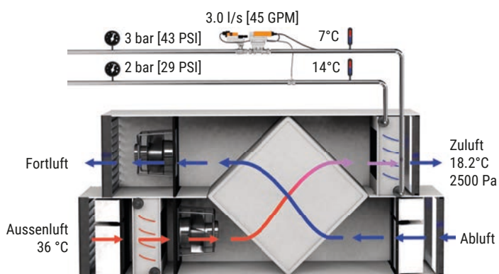
Abb. 55: RLT bei Auslegungsbetrieb.
