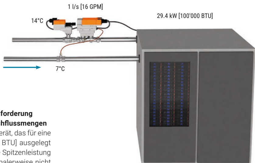
Abb. 111: CRAC-Gerät unter «Auslegungslast-Bedingungen».
