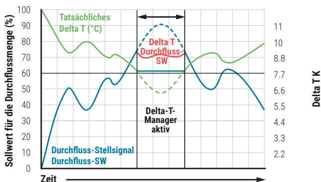
Abb. 32: 'Skalierung Delta-T-Manager' skaliert den Delta-T-Sollwert in Abhängigkeit von der aktuellen Durchflussmenge.
