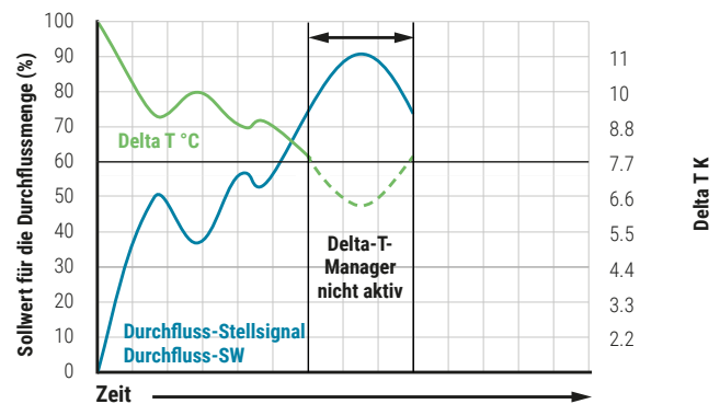
Abb. 29: Wenn der Delta-T-Manager nicht aktiv war, treibt der Durchfluss-Sollwert den Bedarf so hoch, dass das Delta T unter den gewünschten Sollwert von 7.7 K fällt.
