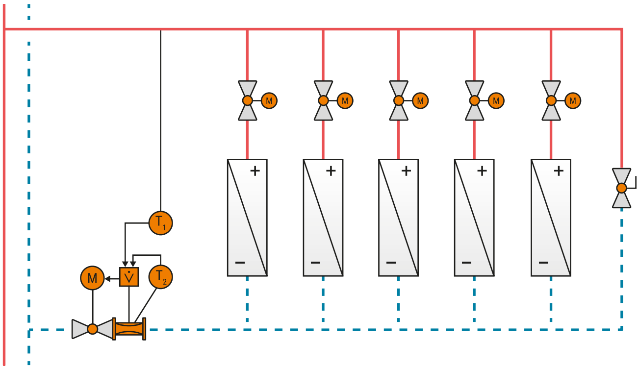
Abb. 101: Eine schematische Darstellung der Installation eines Energieventils in einem Abzweig.
