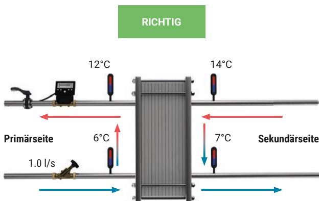
Abb. 66: Typischer Auslegungsdurchfluss (Kühlanwendung).
