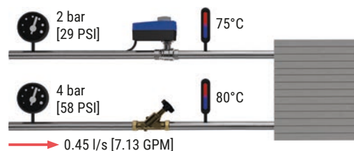
Abb. 98: FCU-Heizbetrieb und Differenzdruckerhöhung.
