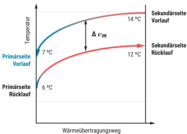
Abb. 67: \Delta v_m mittlere Differenztemperatur bei Auslegungsdurchfluss.
