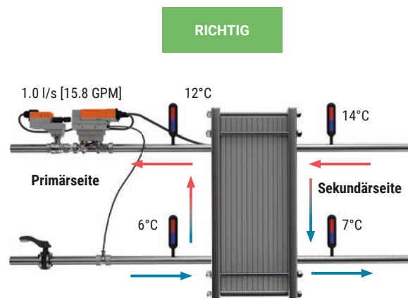
Abb. 71: Dynamischer Abgleich mit Leistungscharakteristik-Überwachung.
