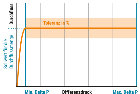
Abb. 24: Regelverhalten im Durchflussregelmodus.
