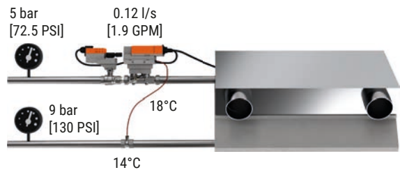
Abb. 91: Kühlbalken mit einem Energieventil.
