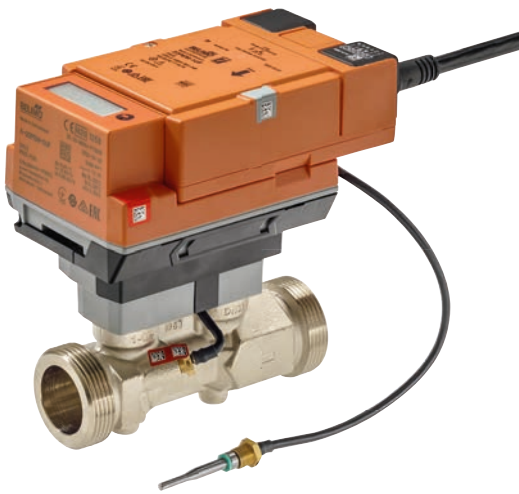
Abb. 41: Thermischer Energiezähler von Belimo.
