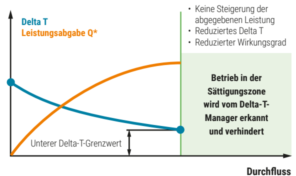
Abb. 95: Der Delta-T-Manager des Energieventils garantiert, dass ein minimales Delta T nicht unterschritten wird.
