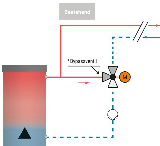
Abb. 116: Kessel mit Hubventil.
