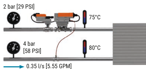
Abb. 99: FCU im Kühlbetrieb, unter Verwendung eines druckunabhängigen EV.
