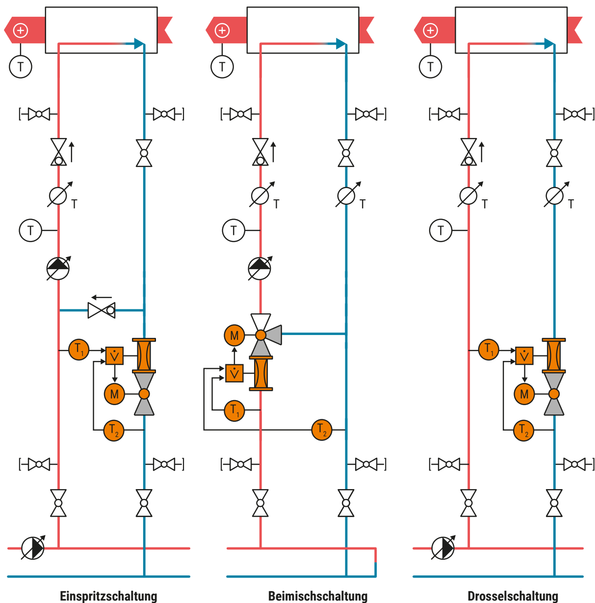
Abb. 118: Ein Überblick über die verschiedenen hydraulischen Grundsaltungen für Heizanwendungen.
