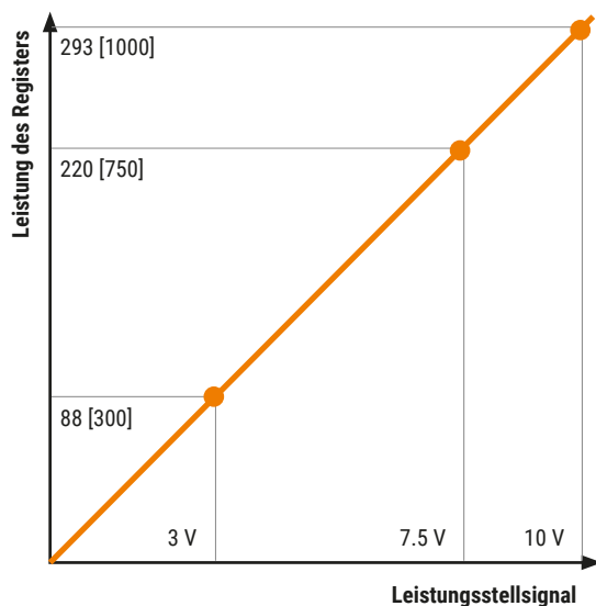
Abb. 27: Beispiel eines Registers im Leistungsregelmodus.
