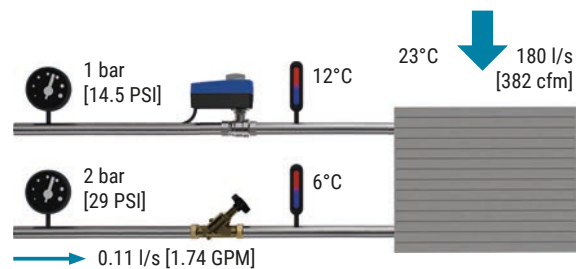
Abb. 76: FCU bei Auslegungsbetrieb.
