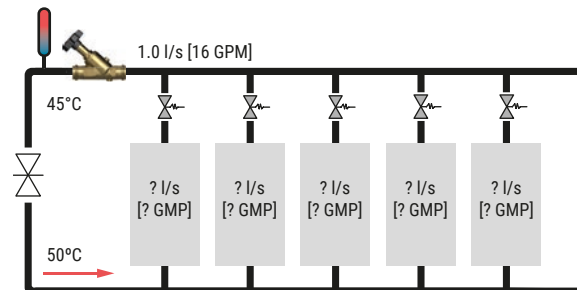
Abb. 102: Mechanische Strangregulierungsventile ermöglichen nur einen statischen Abgleich des Gesamtdurchflusses, wobei die Durchflussmengen zu jeder einzelnen Einheit unbekannt sind.
