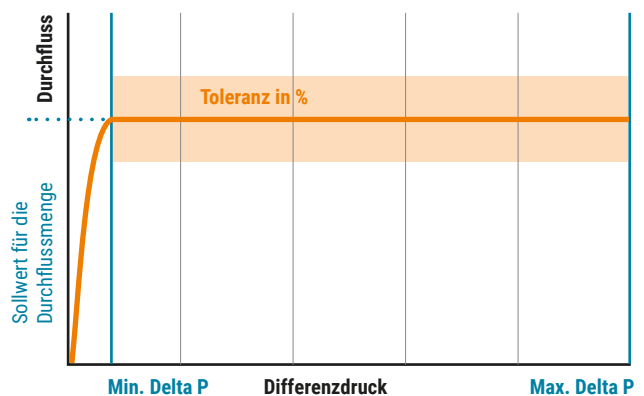
Abb. 50: Der dynamische Abgleich gewährleistet eine genaue Durchflussmenge.
