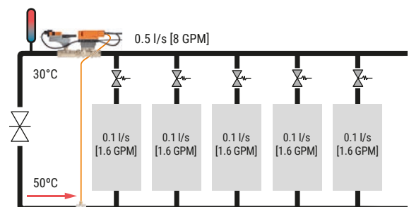
Abb. 103: Mit einem Belimo Energy Valve™ kann der Durchfluss im Abzweig gemessen werden, wenn jedes Ventil geöffnet wird, was eine Überprüfung ermöglicht.
