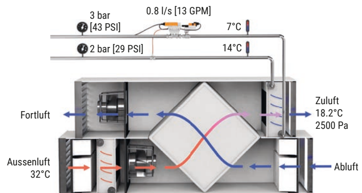
Abb. 57: RLT-Gerät mit Delta-T-optimiertem Durchfluss.
