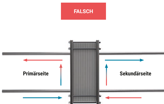
Abb. 62: Kühlungsübergabestation im Gleichstrom angeschlossen.
