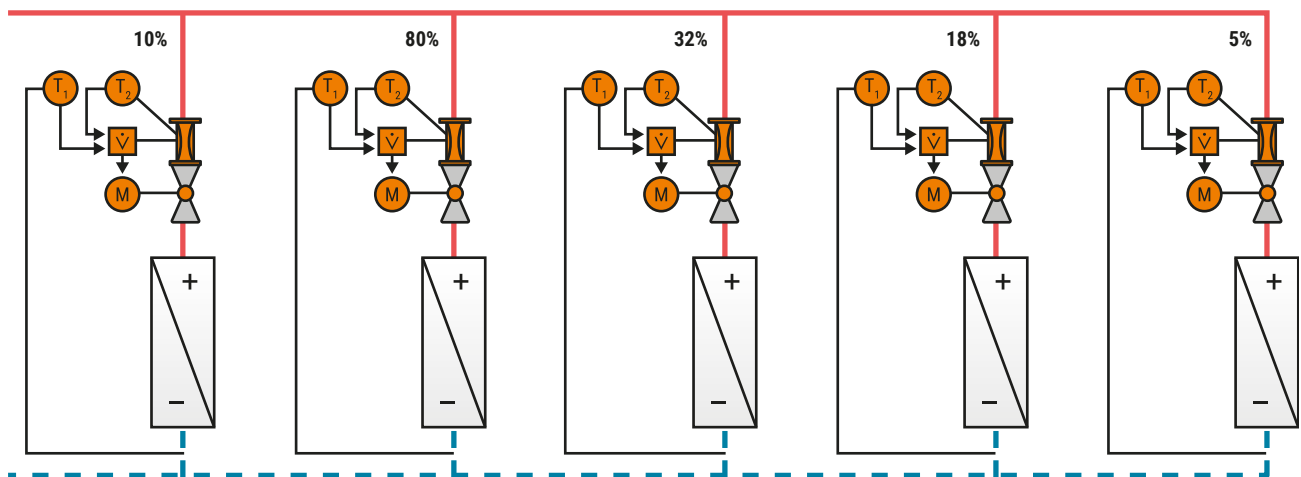
Abb. 45: Die grösste thermische Last befindet sich am Ventil mit der weitesten Öffnung.
