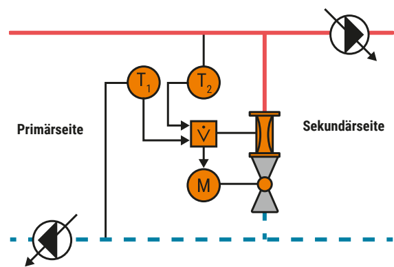
Abb. 47: Ein Energieventil, das die Temperaturspannung des Primärteils und den Durchfluss über die hydraulische Weiche überwacht.
