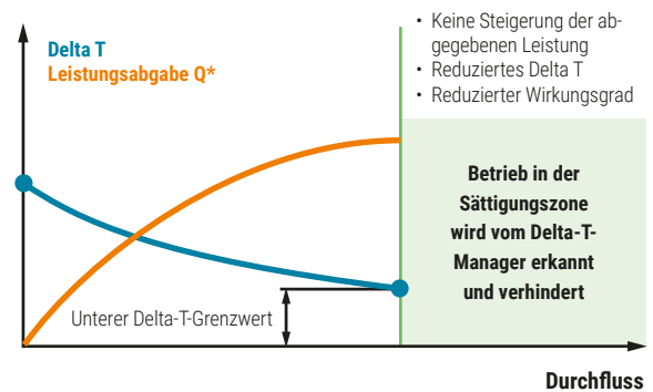
Abb. 52: Verbesserte Energieeffizienz mit dem aktivierten Delta-T-Manager der Energieventile.
