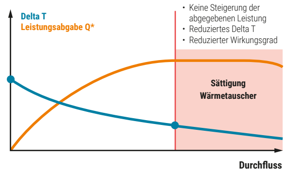
Abb. 94: Niedriges Delta T an einem Verbraucher (z.B. Gebläsekonvektor).
