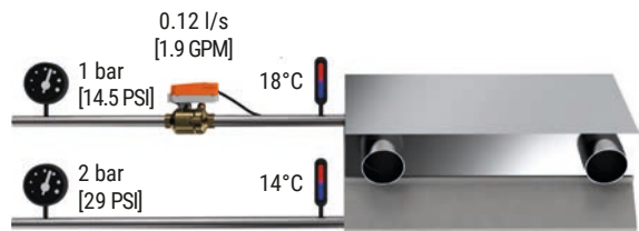
Abb. 90: Kühlbalken mit einem mechanischen PI-Ventil.
