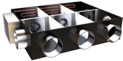
Abb. 73: Gebläsekonvektor
