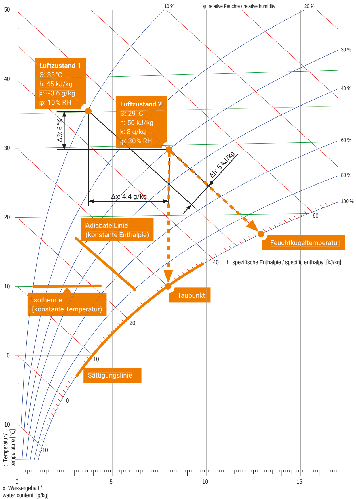
Abb. 88: Der Taupunkt hängt von der Lufttemperatur und der Luftfeuchtigkeit ab.
