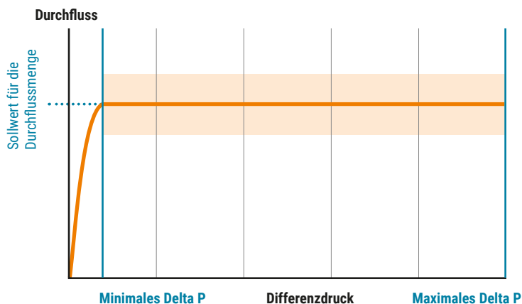
Abb. 11: Verbesserte Stabilität mit mechanischen PI-Ventilen.
