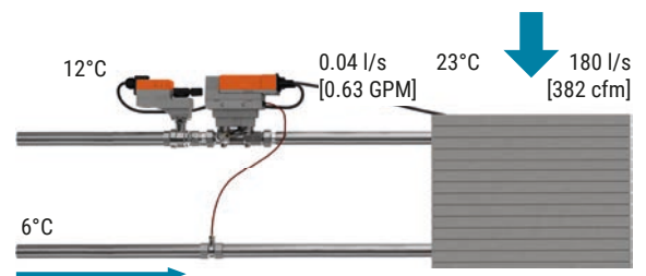
Abb. 80: FCU mit Delta-T-optimiertem Ventildurchfluss.
