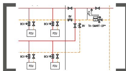
Heizungsanlage - Differenzdruckregelung
