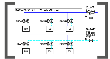
Kühlanlage - Zonenventil
