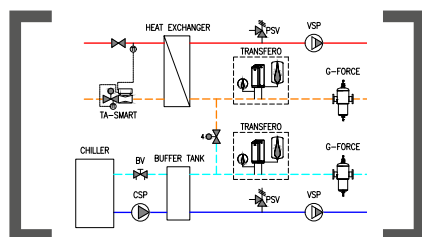
4-Leiter-System - Zonenventil
