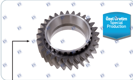
3. VİTES DİŞLİSİ
