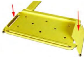
Abfallsicherungen vorne und hinten an den Radaufnahmeplatten
