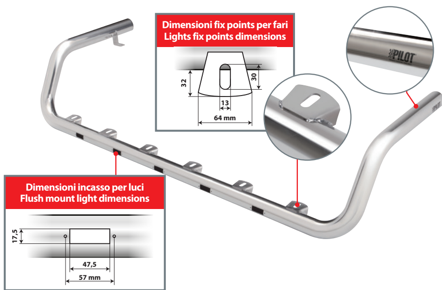
BARRE PER TETTO ROOF BARS
