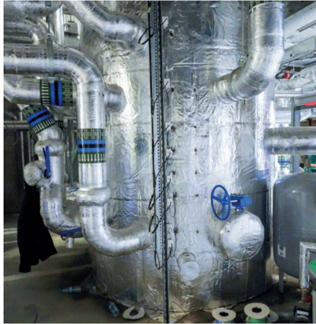
Zortström Multi-PG-H, 3-stufig (Heizung) Durchmesser 2.000 mm
