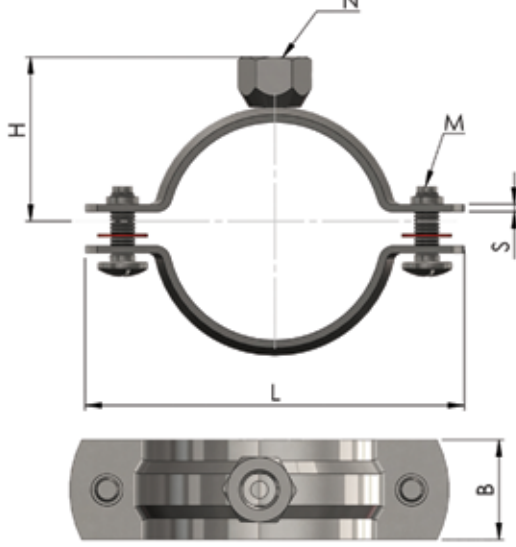
Lastiksiz sıkma ölçüsü / Clamping range without rubber
