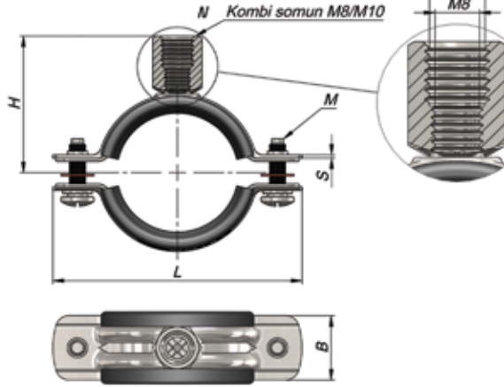
Lastiksiz sıkma ölçüsü / Clamping range without rubber
