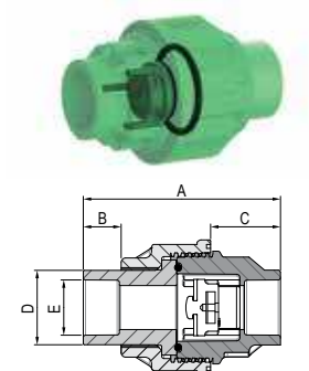
BOCCHETTONE IN PP-RCT con valvola di non ritorno saldatura a bicchiere PP-RCT PIPE UNION with check valve socket welding
