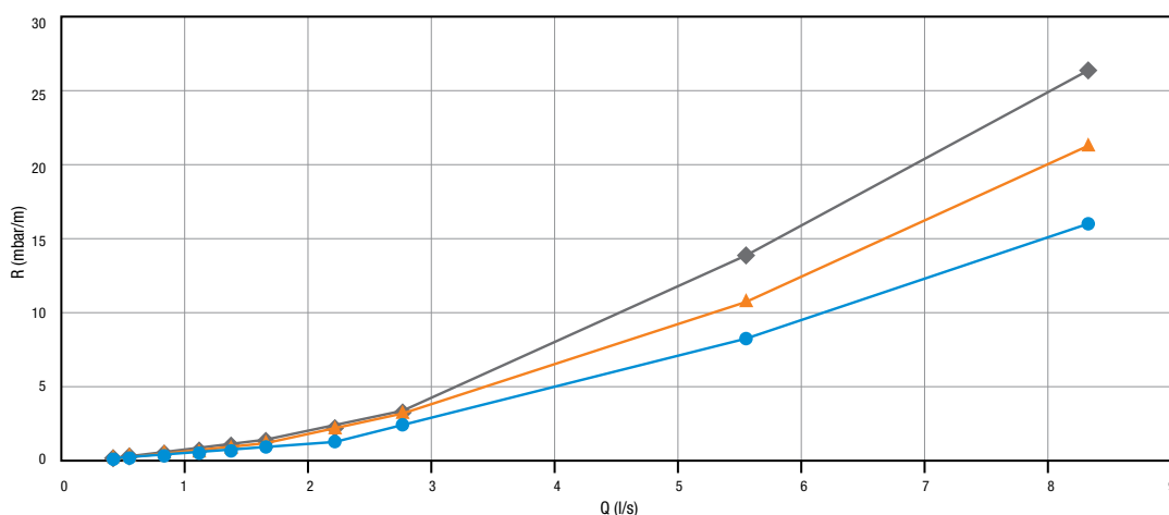
Confronto perdite di carico tubazioni Ø 50 mm, T 50°C Comparison between pressure drops of pipes Ø 50 mm, T 50°C
