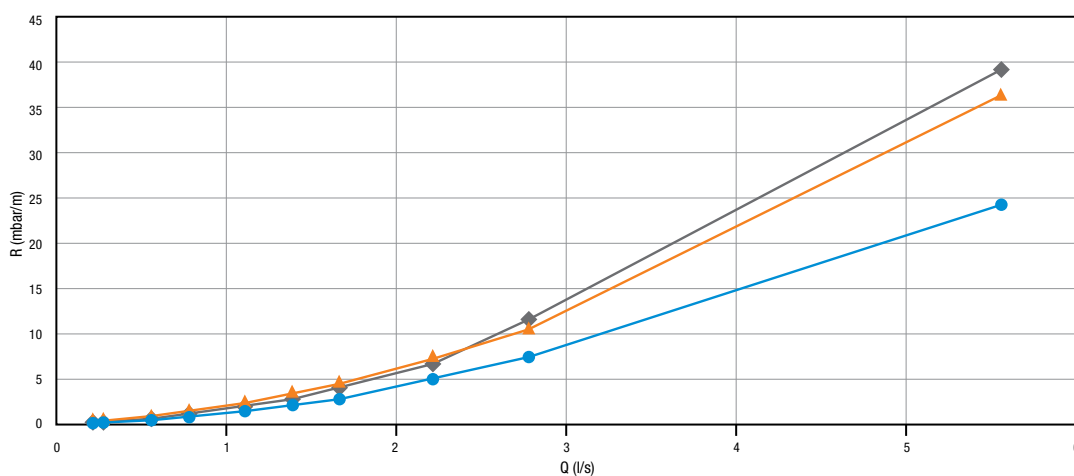
Confronto perdite di carico tubazioni Ø 40 mm, T 50°C Comparison between pressure drops of pipes Ø 40 mm, T 50°C
