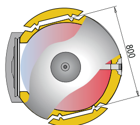
Detailansicht der abnehmbaren Dämmseite bei 800 und 1000 Liter Speichern für Montageöffnungen ab 800 mm
