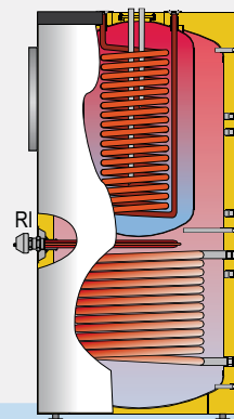
Elektrische Zuheizung in Speichern der Serie CORAL VITRO "DOPPELMANTEL"
