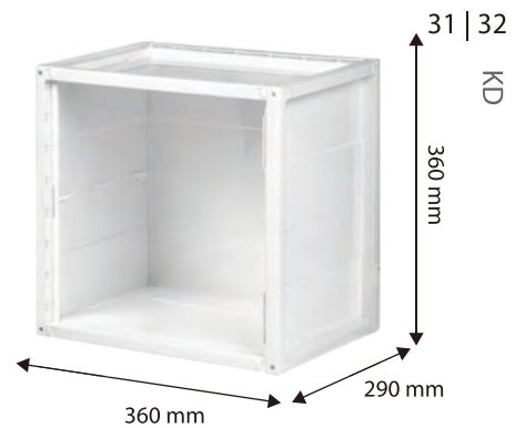
KD-2936 360W x 290D x 360H mm
