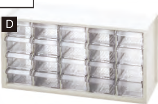
A9-520 378W x 154D x 192H mm
