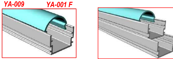
ALM. ve PC.DİFÜZÖR 610 cm
