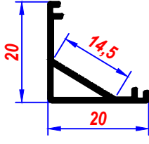
L KÖŞE Profili 12-14 mm lik PCB ye uygun
