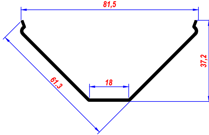
ALM.PROF.-PC DİFÜZÖR 610 cm
