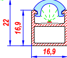
MONTAJ AVZ-001 PS
