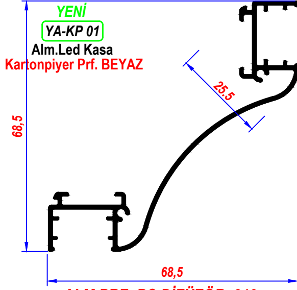
ALM.PRF.-PC DİFÜZÖR 610 cm
