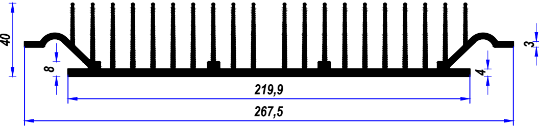
ADS - 267 Alm. Sğt. Prf. Ölçek 1/2
