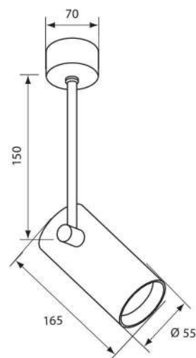
SP709 BK LUX
