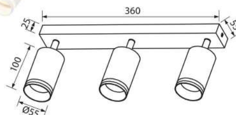
SP733-3L WH KING
