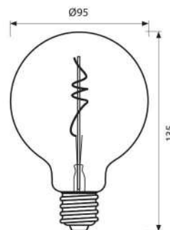
GFD95 4W E27
