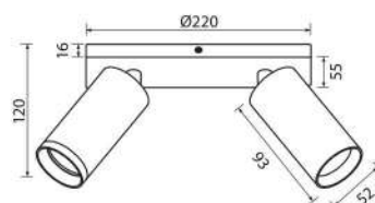
SP712-2L WH LUX
