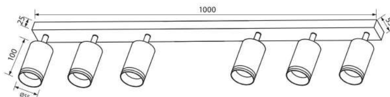
SP736-6L WH KING
