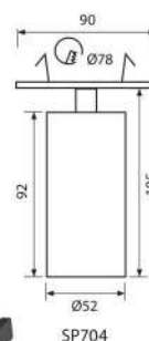
SP704 WH LUX
