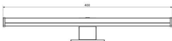
ARMI LED за монтаж над горен шкаф / ARMI LED for over cabinet mounting
