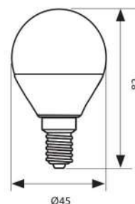
MGL E14 MAX LED
