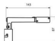
ARMI LED за монтаж на стена / ARMI LED for wall mounting
