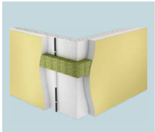
Brandschutzbandage zur Verhinderung der Brandübertragung über isCon® im WDVS
