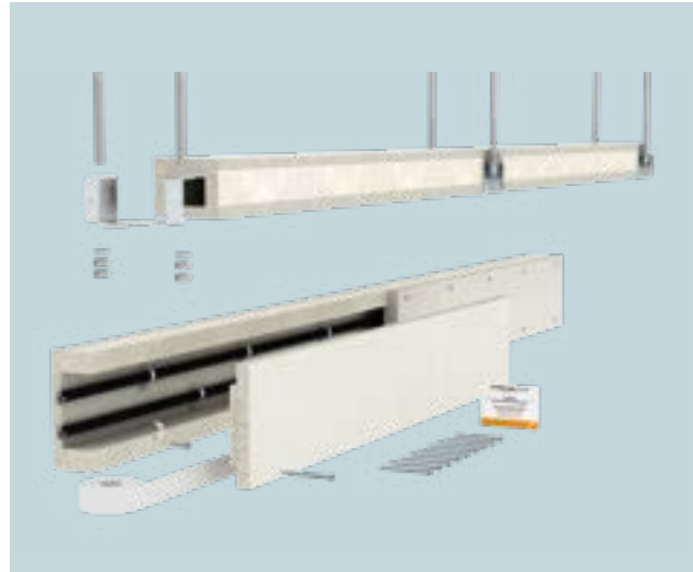
Brandschutzkanäle PYROLINE® Sun PV zur Leitungsverlegung in Flucht- und Rettungswegen
