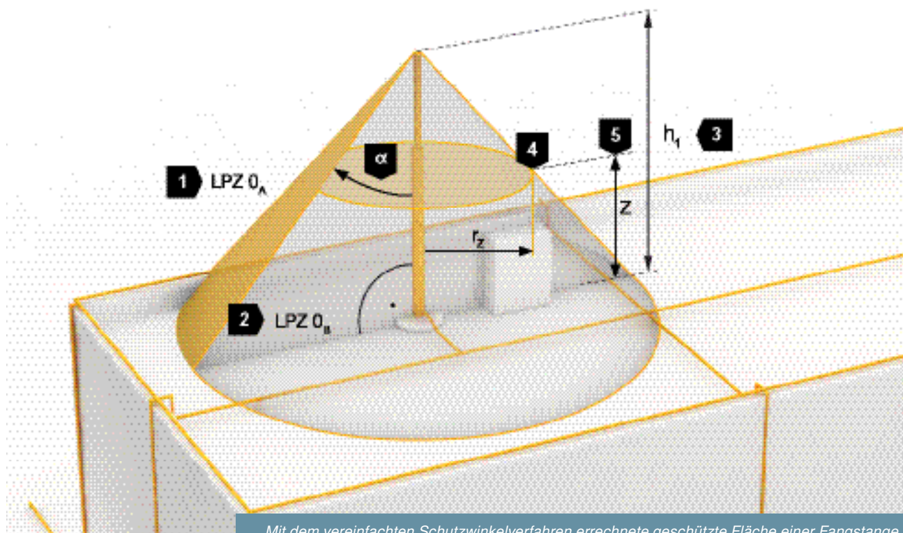
Mit dem vereinfachten Schutzwinkelverfahren errechnete geschützte Fläche einer Fangstange
