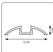
ΠΡΟΦΙΛ ΕΞΩΤΕΡΙΚΟ ΟΒΑΛ PROFILE EXTERNAL SINGLE OVAL
