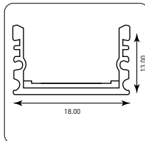
ΠΡΟΦΙΛ ΕΞΩΤΕΡΙΚΟ PROFILE EXTERNAL SINGLE
