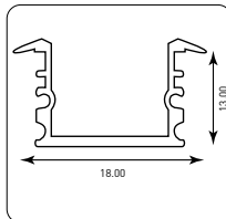
ΠΡΟΦΙΛ ΧΩΝΕΥΤΟ PROFILE RECESSED SINGLE
