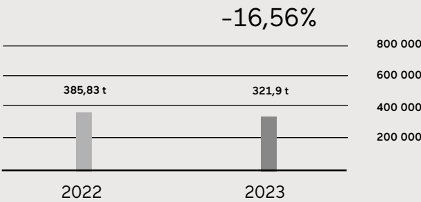
Gesamtabfallaufkommen (Tonnen)
