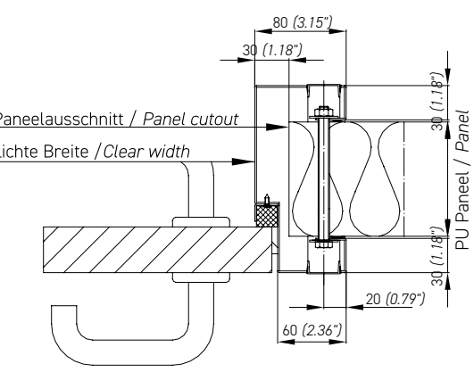
Abb. 1.1 Klemmrahmen (Schlossseite) Fig. 1.1 Clamping frame (Lock side)
