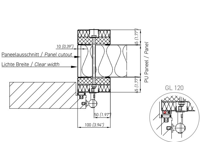
Abb. 3.3 Klemmrahmen Fig. 3.3 Clamping frame
