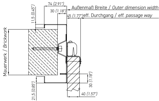
Abb. 4.2 Klemmrahmen, U-Zarge geteilt Fig. 4.2 U-frame, divided
