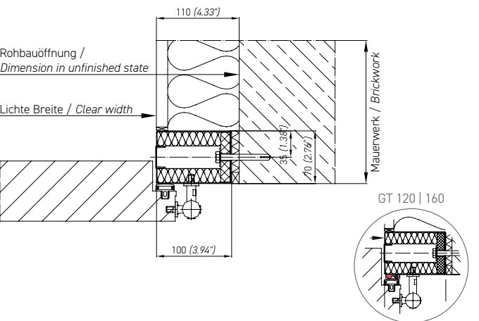
Abb. 2.4 Blockrahmen 100x70 mm (Sacklöcher im Leibrungsbereich) Fig. 2.4 Block frame 3.94"x 2.76" (Pocket holes in the reveal area)
