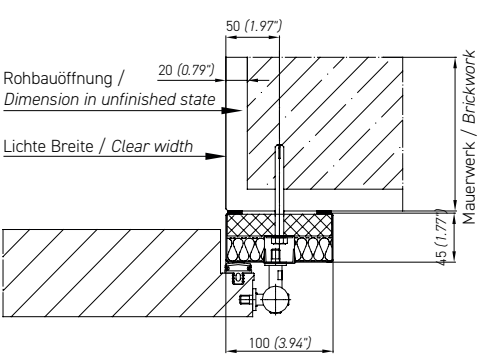
Abb. 3.2 Flachrahmen 100x45 mm (mit Sacklöchern) Fig. 3.2 Flat frame 3.94"x1.77" (with pocket holes)
