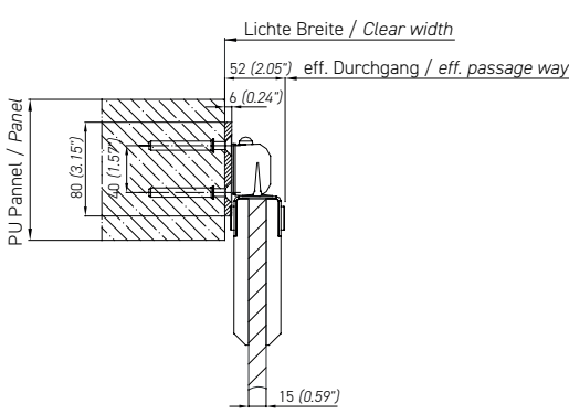
Abb. 4.6 MW-Flach-Pofil Fig. 4.6 Brickwork frame
