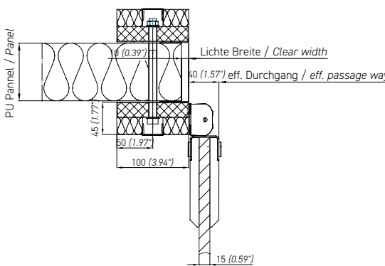
Abb. 4.5 Klemmrahmen Fig. 4.5 Clamping frame
