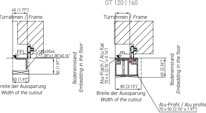
Abb. 2.6 / 2.7 Schwelleneinbau Fig. 2.6 / 2.7 Threshold installation
