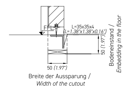
Abb. 1.6 Schwelleneinbau Fig. 1.6 Threshold installation
