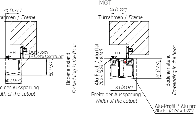
Abb. 2.6 / 2.7 Schwelleneinbau Fig. 2.6 / 2.7 Threshold installation
