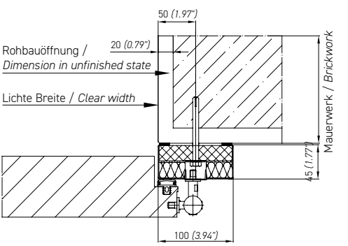
Abb. 2.2 Flachrahmen 100x45 mm (mit Sacklöchern) Fig. 2.2 Flat frame 3.94"x 1.77" (with pocket holes)
