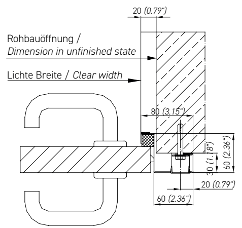
Abb. 1.4 Mauerwerksrahmen / Eckzarge (Schlossseite) Fig. 1.4 Brickwork frame / Corner frame (Lock side)
