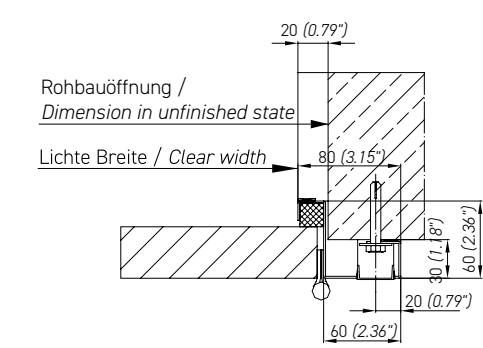
Abb. 1.5 Mauerwerksrahmen (Bandseite) Fig. 1.5 Brickwork frame (Hinge side)
