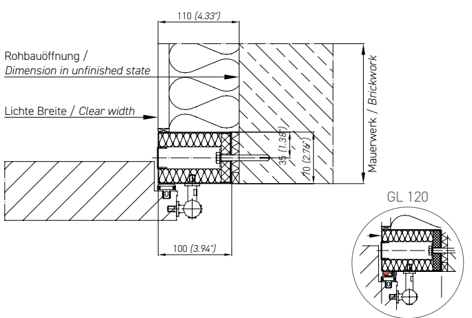
Abb. 3.4 Blockrahmen 100x70 mm (Sacklöcher im Leibungsbereich) Fig. 3.4 Block frame 3.94"x2.76" (Pocket holes in the reveal area)
