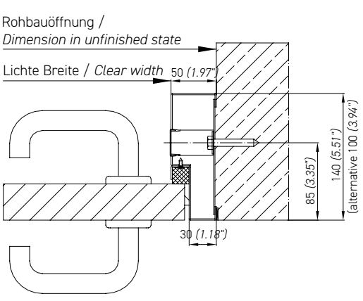
Abb. 1.3 Mauerwerksrahmen / Blockrahmen Fig. 1.3 Brickwork frame / Block frame
