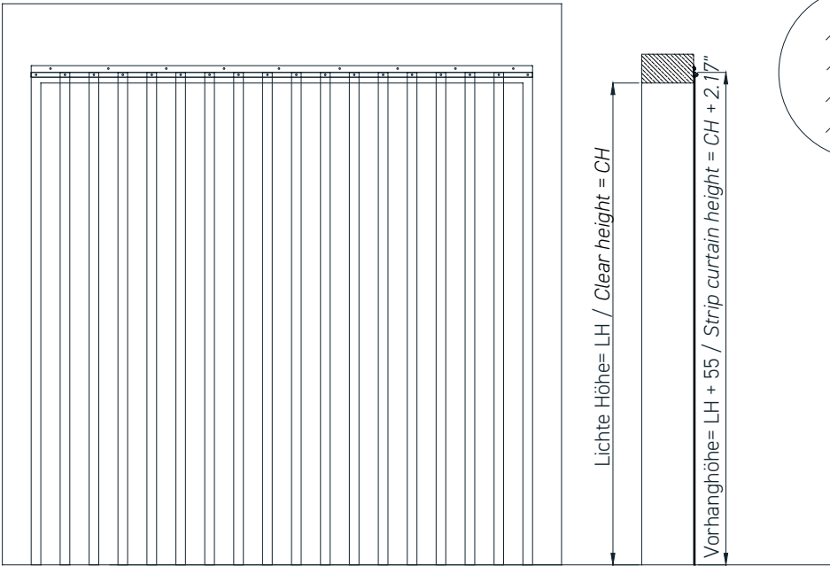
Vorsturzmontage / Wall assembly
