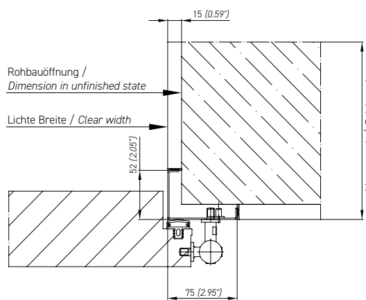
Abb. 2.3 Eckzarge (mit Mauerwerksanker) Fig. 2.3 Corner frame (with brickwork anchor)
