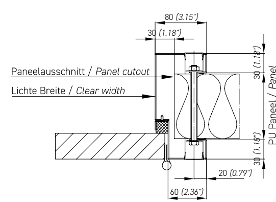
Abb. 1.2 Klemmrahmen (Bandseite) Fig. 1.2 Clamping frame (Hinge side)
