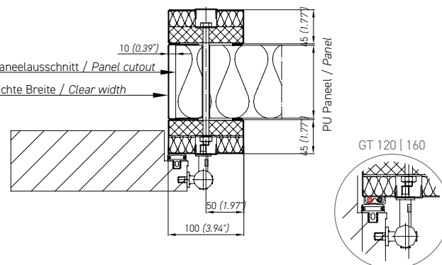
Abb. 2.5 Klemmrahmen Fig. 2.5 Clamping frame
