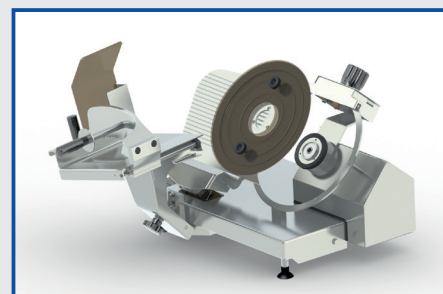
BLADE EXTRACTOR EXTRACTEUR LAME EXTRACTOR CUCHILLA MESSER EXTRACTOR
