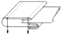
F8759 散底落樸褲頭筒(底有捆邊)
