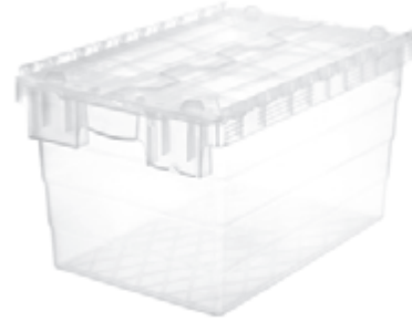
HP-6435-MK SF En/W Boy/L Yükseklik Dış / Ext 400 x 600 x 360 mm İç / Int 365 x 545 x 347 mm
