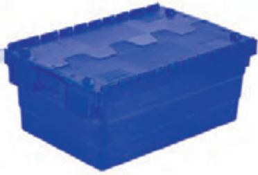
HP-6425-MK En/W Boy/L Yükseklik Dış / Ext 400 x 600 x 250 mm İç / Int 365 x 543 x 232 mm
