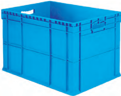
Kod / Code HP-4003 En/W Boy/L Yükseklik Dış / Ext 400 x 600 x 400 mm İç / Int 365 x 565 x 386 mm
