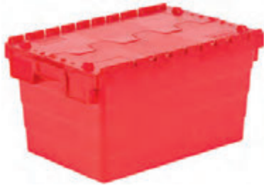
HP-6432-MK En/W Boy/L Yükseklik Dış / Ext 400 x 600 x 320 mm İç / Int 365 x 545 x 302 mm
