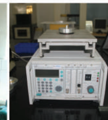
油封緊迫力測試機 Radial Force Tester
