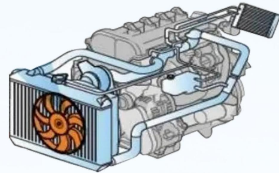
电子扇/Radiator Fan
