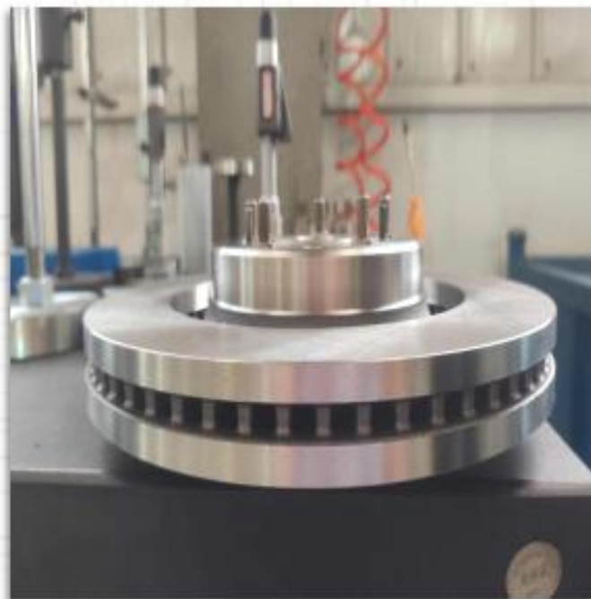
位置度检具 Position gauge
