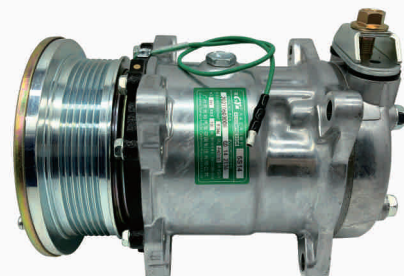
型号 / MODEL: 5S14 编码 / PART NO.: GD.14.2136
