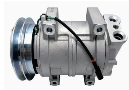
型号 / MODEL: DKS15 编码 / PART NO.: GT.15.210
