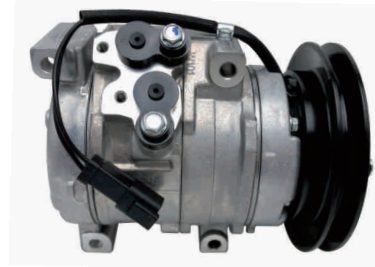
型号 / MODEL: 10S15C 编码 / PART NO.: GS.15.801
