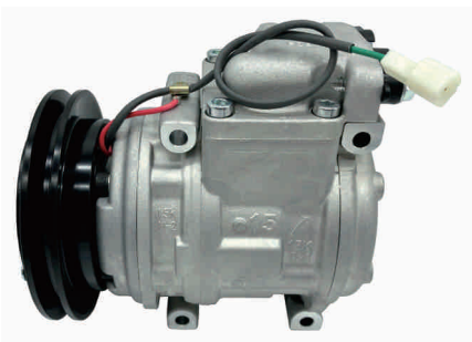
型号 / MODEL: 10PA15C 编码 / PART NO.: GP.15.2403
