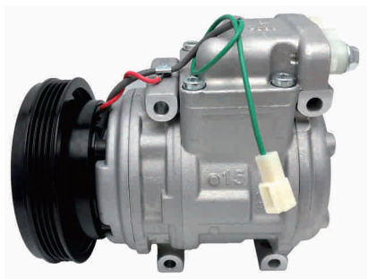
型号 / MODEL: 10PA15C 编码 / PART NO.: GP.15.1601
