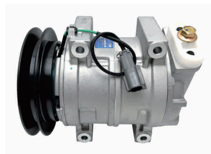
型号 / MODEL: DKS15 编码 / PART NO.: GT.15.1403
