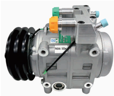
型号 / MODEL: GY10P35C 编码 / PART NO.: GP.38.501
