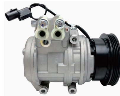
型号 / MODEL: 10PA15C 编码 / PART NO.: GP.15.301
