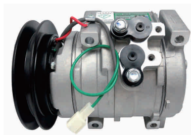
型号 / MODEL: 10S15C 编码 / PART NO.: GS.15.201
