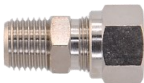
RACCORDO CON OGIVA DRITTO MASCHIO CONICO IN OTTONE NICHELATO
