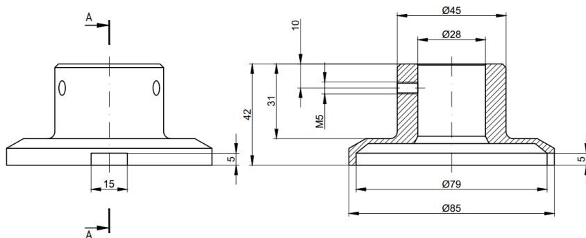
PRESEK "A" - "A"
