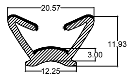
Die No. : 10240 Wt/mtr : 100 gm/mtr
