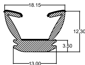
Die No. : 10404 Wt/mtr : 92 gm/mtr
