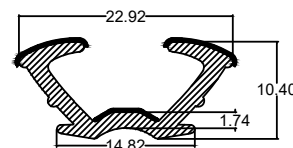
Die No. : 10107 Wt/mtr : 92 gm/mtr
