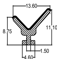
Die No. : 10441 Wt/mtr : 50 gm/mtr
