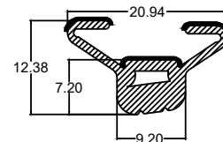
Die No. : 10046 Wt/mtr : 96 gm/mtr
