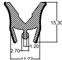
Die No. : 10234 Wt/mtr : 114 gm/mtr
