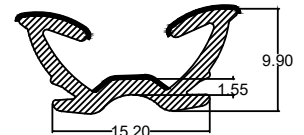
Die No. : 10006 Wt/mtr : 113 gm/mtr
