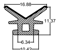
Die No. : 10278 Wt/mtr : 90 gm/mtr
