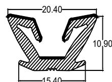
Die No. : 10446 Wt/mtr : 40 gm/mtr
