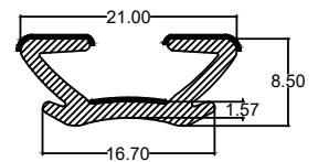
Die No. : 10023 Wt/mtr : 89 gm/mtr
