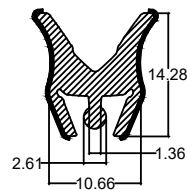
Die No. : 10198 Wt/mtr : 100 gm/mtr
