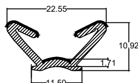
Die No. : 10106 Wt/mtr : 82 gm/mtr
