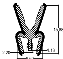
Die No. : 10094 Wt/mtr : 90 gm/mtr
