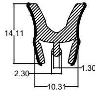
Die No. : 10254 Wt/mtr : 106 gm/mtr
