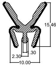
Die No. : 10003 Wt/mtr : 86 gm/mtr
