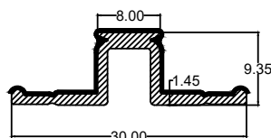
Die No. : 10403 Wt/mtr : 80 gm/mtr
