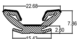
Die No. : 10423 Wt/mtr : 120 gm/mtr
