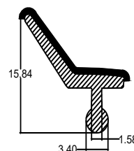
Die No. : 10051 Wt/mtr : 63 gm/mtr
