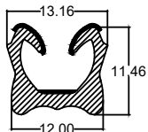
Die No. : 10241 Wt/mtr : 98 gm/mtr
