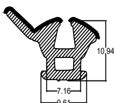
Die No. : 10223 Wt/mtr : 190 gm/mtr
