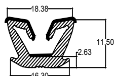
Die No. : 10204 Wt/mtr : 135 gm/mtr
