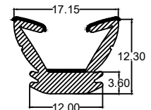
Die No. : 10372 Wt/mtr : 100 gm/mtr
