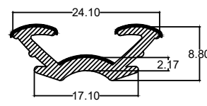
Die No. : 10093 Wt/mtr : 95 gm/mtr
