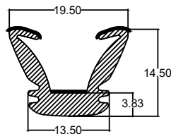
Die No. : 10016 Wt/mtr : 134 gm/mtr
