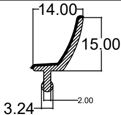
Die No. : 10025 Wt/mtr : 76 gm/mtr
