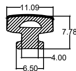
Die No. : 10354 Wt/mtr : 71 gm/mtr
