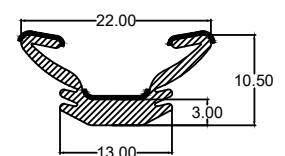
Die No. : 10406 Wt/mtr : 92 gm/mtr
