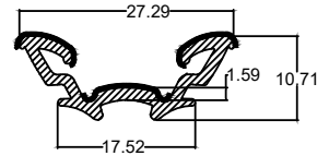
Die No. : 10159 Wt/mtr : 100 gm/mtr
