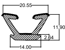
Die No. : 10186 Wt/mtr : 112 gm/mtr
