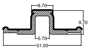
Die No. : 10007 Wt/mtr : 87 gm/mtr
