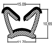
Die No. : 10002 Wt/mtr : 82 gm/mtr
