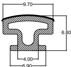
Die No. : 10386 Wt/mtr : 50 gm/mtr
