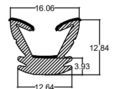
Die No. : 10096 Wt/mtr : 128 gm/mtr
