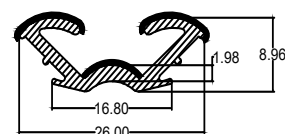
Die No. : 10454 Wt/mtr : 103 gm/mtr
