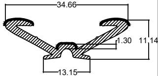
Die No. : 10110 Wt/mtr : 132 gm/mtr
