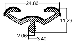
Die No. : 10155 Wt/mtr : 97 gm/mtr
