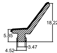
Die No. : 10277 Wt/mtr : 76 gm/mtr
