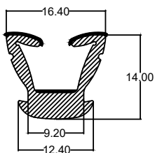
Die No. : 10279 Wt/mtr : 110 gm/mtr
