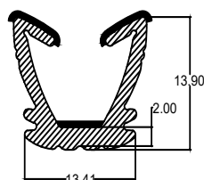
Die No. : 10285 Wt/mtr : 86 gm/mtr
