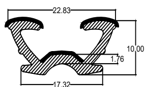
Die No. : 10071 Wt/mtr : 110 gm/mtr
