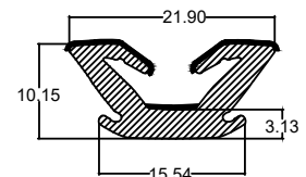
Die No. : 10108 Wt/mtr : 138 gm/mtr
