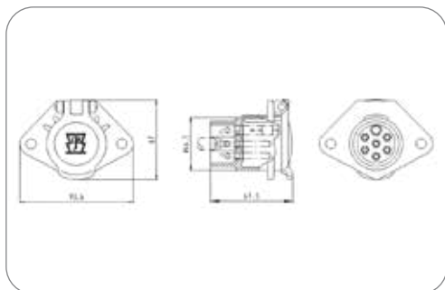
7P/24V Steckdose (ISO 3731 - Typ S) 7P/24V Socket (ISO 3731 - Type S)
