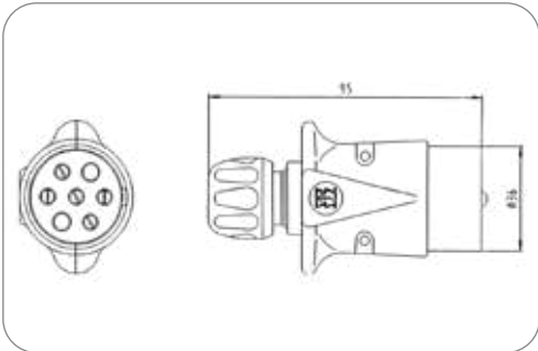
7P/12V Stecker (ISO 3732 - Typ S) 7P/12V Plug (ISO 3732 - Type S)
