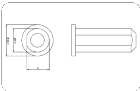
"JAEGER Basic" Anschlaghülse für 7P/12V/24V und 15P/24V (ISO 7638-1 / ISO 7638-2 / ISO 25981 / ISO 12098) Kontaktstifte "JAEGER Basic" Stopper bush for 7P/12V/24V and 15P/24V (ISO 7638-1 / ISO 7638-2 / ISO 25981 / ISO 12098) contact pins
