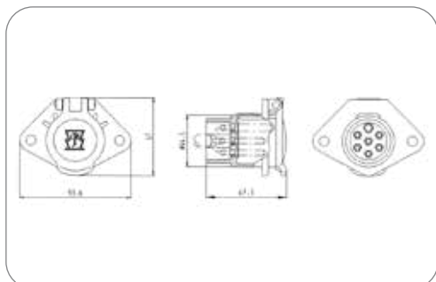
7P/24V Steckdose (ISO 1185 - Typ N) 7P/24V Socket (ISO 1185 - Type N)
