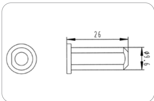
Anschlaghülse für 7P/12V (ISO 1724 und ISO 3732) Kontaktstifte Stopper bush for 7P/12V (ISO 1724 und ISO 3732) contact pins
