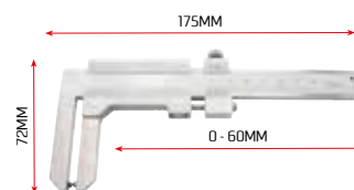
#47024 Edelstahlmessschieber für Scheibenbremsen
