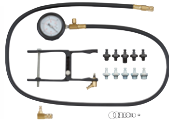
#818011 Öldruck-Test-Satz im Koffer
