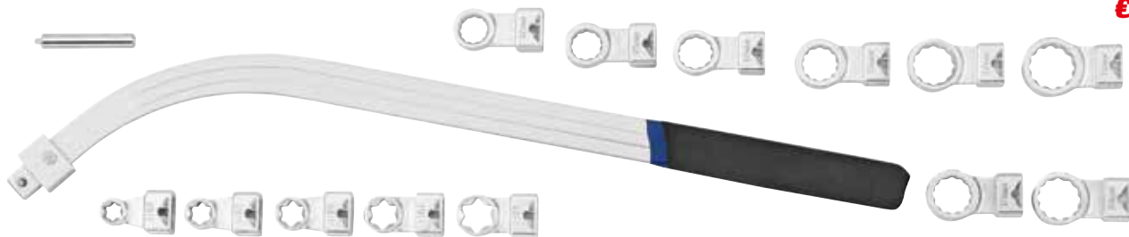
#805015 Keilriemen Schlüssel Gegenhalter TX und 12-kant, 15-tlg. Speziell zum Auswechseln und Spannen von Spann- und Laufrollen. Satz beinhaltet: - 8 12-kant Einsteckensätze - 12-19mm - 5 Einsteckensätze TX E10-E18 - 1 gebogener Einsteckhalter
