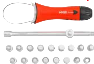
#302001 1/2" Ölablassschrauben- und Filter-Satz 20-tlg.
