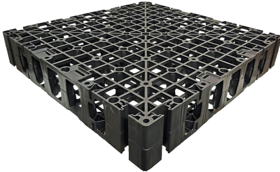
Variobox 75 N mit 600 x 600 x 75 mm
