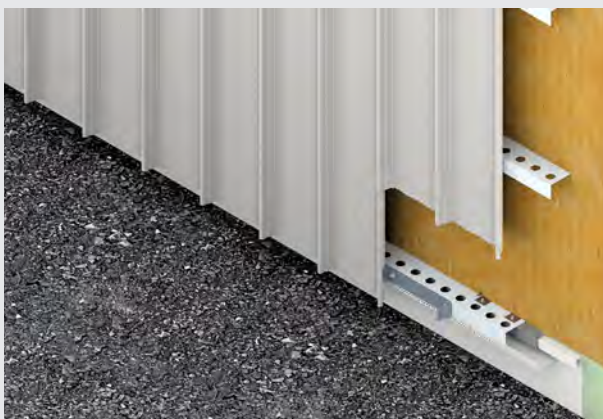
Unterer Fassadenabschluss – senkrecht mit Gleitbügel auf Betonwand mit Dämmung
