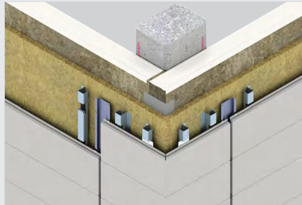
Außenecke als ECKelement – Planum waagrecht auf Kassetten-Innenschale mit vorgesetzter Dämmung
