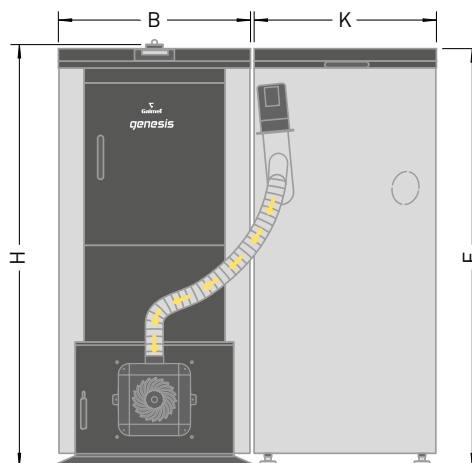
scheme - Genesis Plus KPP 25÷34 kW
