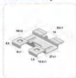
TFM Bend Clip
