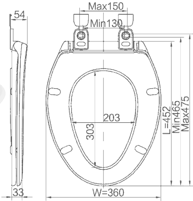
安装尺寸：465-475*130-150
