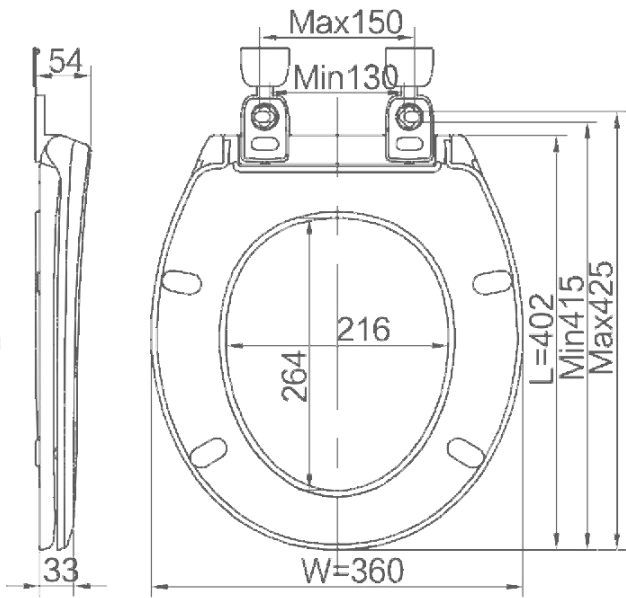
安装尺寸：415-425*130-150
